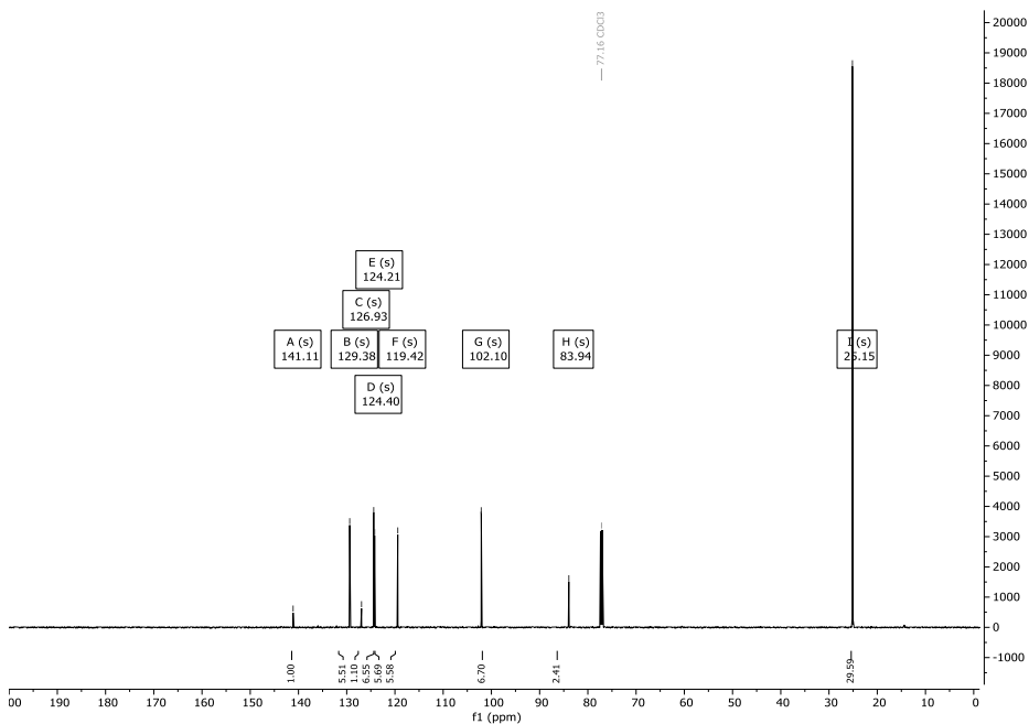
Abbildung 143: 13 C-NMR-Spektrum (151 MHz) von Verbindung 38 in CDCl 3 .
