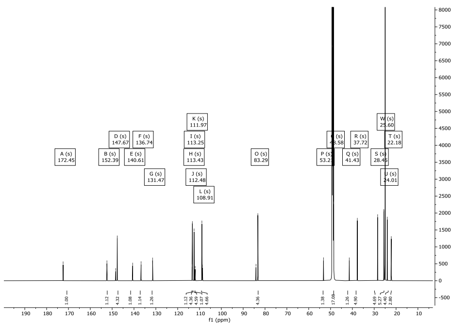
Abbildung 248: Synthetisches ^{13}\text{C} -NMR-Spektrum (176 MHz) des prädominanten Rotamers von Verbindung 204 in \text{CD}_3\text{OD} .
