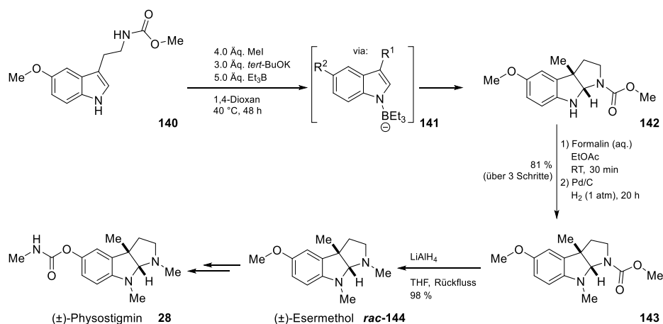
Schema 23: Biomimetischer Ansatz zur Synthese von (±)-Esermethol ( rac-144 ) ausgehend von Tryptamincarbamat 140 mithilfe einer dearomatisierenden Zyklisierung nach You et al. [180]
