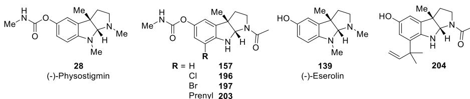
Abbildung 48: Chemische Struktur der Pyrroloindolcarbamate 157 , 196 , 197 und 204 sowie der Naturstoffe 28 und 139 , deren IC_{50} anhand des Ellmans-Assays bestimmt wurden.
