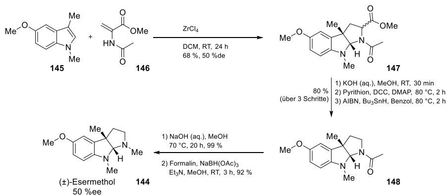
Schema 24: Synthese von (±)-Esermethol ( 144 ) ausgehend von N -3-Methyl-5-Methoxyindol ( 145 ) über eine Lewis-Säure-vermittelte [2+3]-Cycloaddition mit Verbindung 146 nach Spadoni et al. [182]
