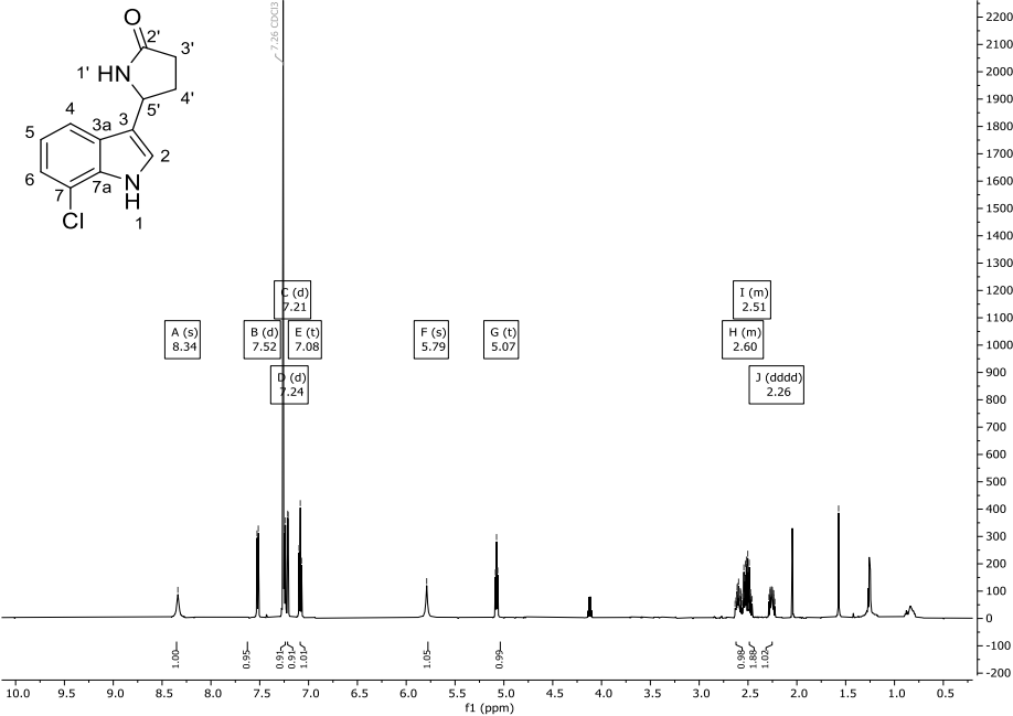
Abbildung 152: ^1\text{H} -NMR-Spektrum (600 MHz) von Verbindung 88 in \text{CDCl}_3 .
