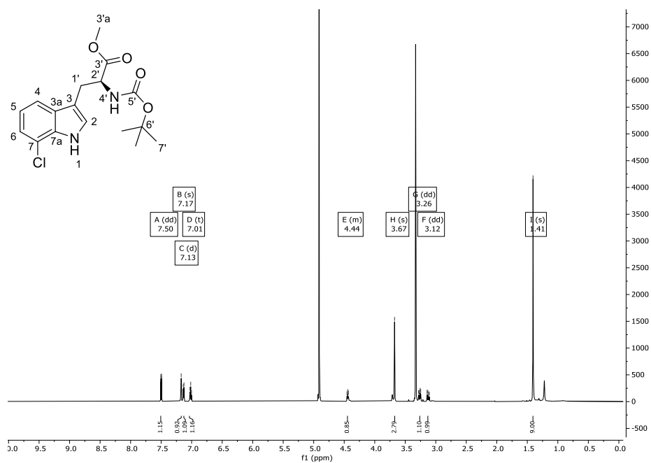
Abbildung 102: ^1\text{H} -NMR-Spektrum (600 MHz) von Verbindung 103 in \text{CD}_3\text{OD} .
