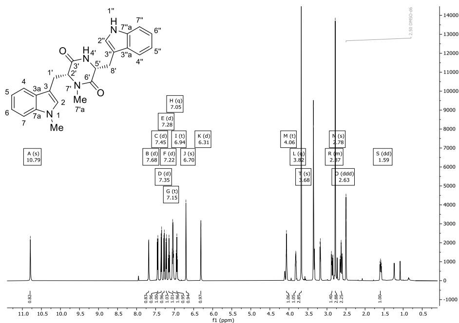
Abbildung 273: 1 H-NMR-Spektrum (600 MHz) von Verbindung 347 in d 6 -DMSO.
