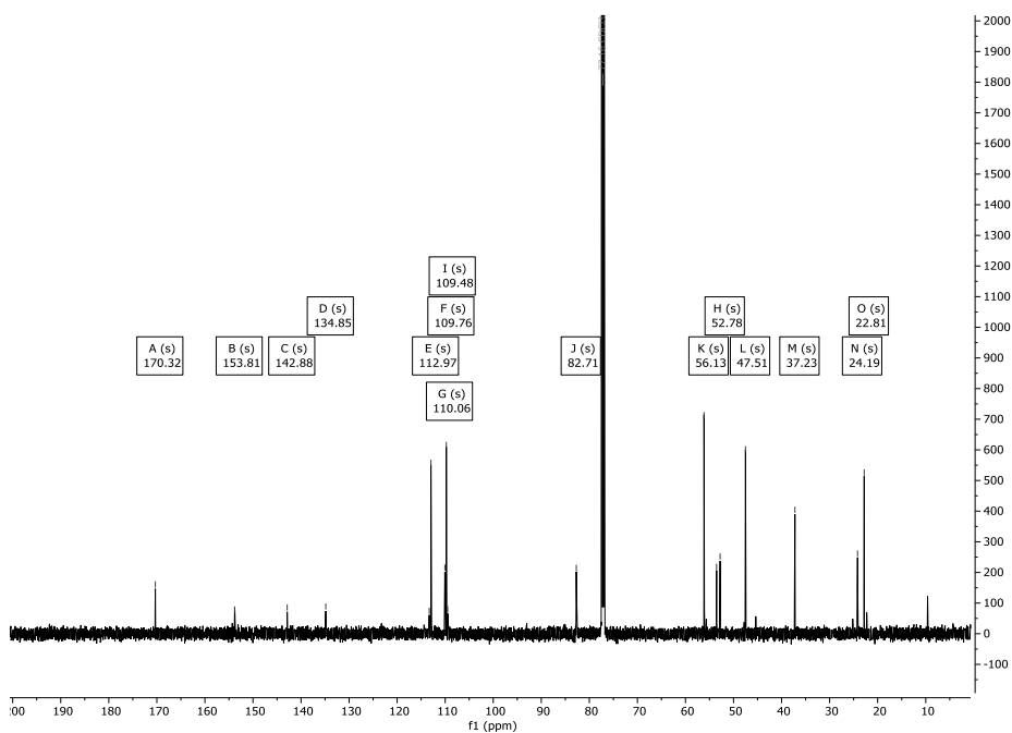
Abbildung 228: ^{13}\text{C} -NMR-Spektrum (151 MHz) von Verbindung rac -200 in \text{CDCl}_3 .
