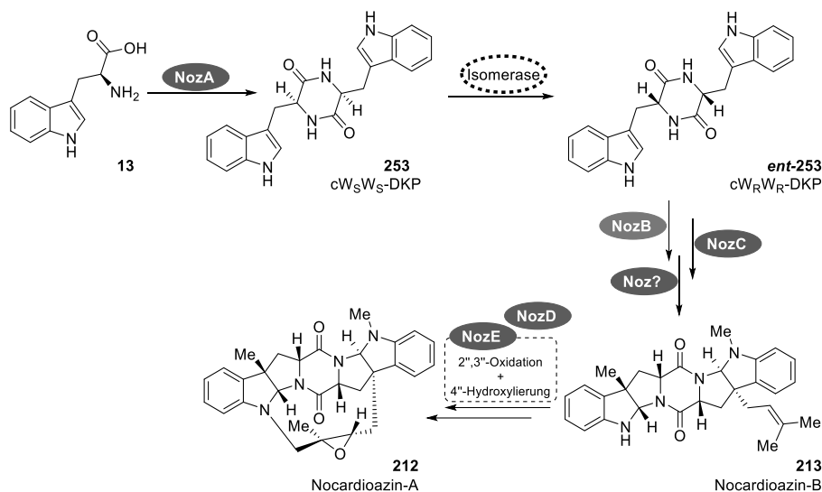
Schema 46: Vermutete Biosynthese von Nocardioazin-A und -B ( 212 und 213 ) nach Viswanathan et al. katalysiert durch den noz -Gencluster. [226]
