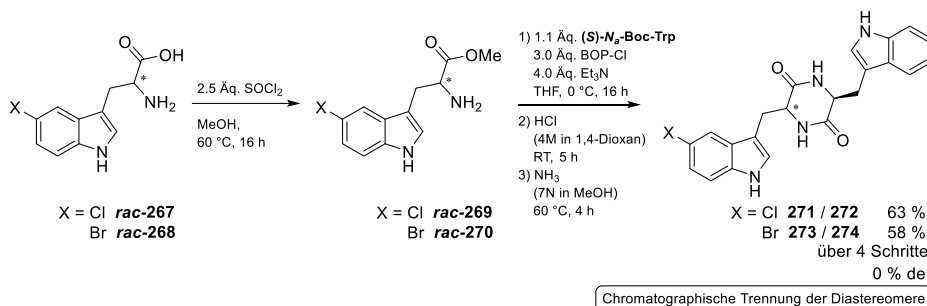
Schema 52: Synthese des ( S,S )-konfigurierten 5-Chlor- und 5-Brom-cWW-DKP 271 und 273 ausgehend von einem racemischen Gemisch der halogenierten Tryptophane über eine Veresterung, Peptidknüpfung und anschließende Entschützung der verwendeten PGs.
