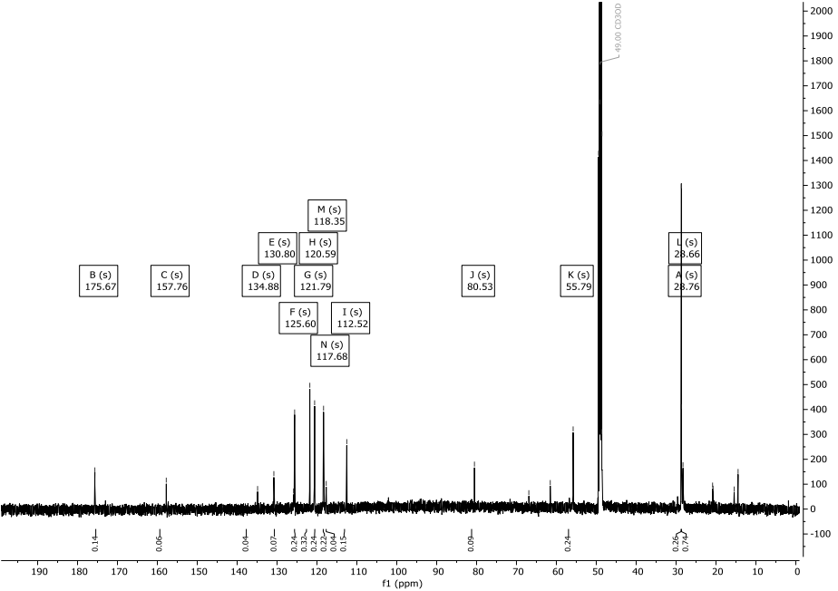
Abbildung 117: ^{13}\text{C} -NMR-Spektrum (151 MHz) von Verbindung 105 in \text{CD}_3\text{OD} .
