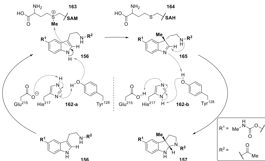
Schema 28: Anhand der Kristallstruktur vermuteter Reaktionsmechanismus der Methyltransferase PsmD mit katalytischer Triade, bestehend aus Glutamat 215 , Histidin 217 und Tyrosin 128 , nach D. Amariei. [59]
