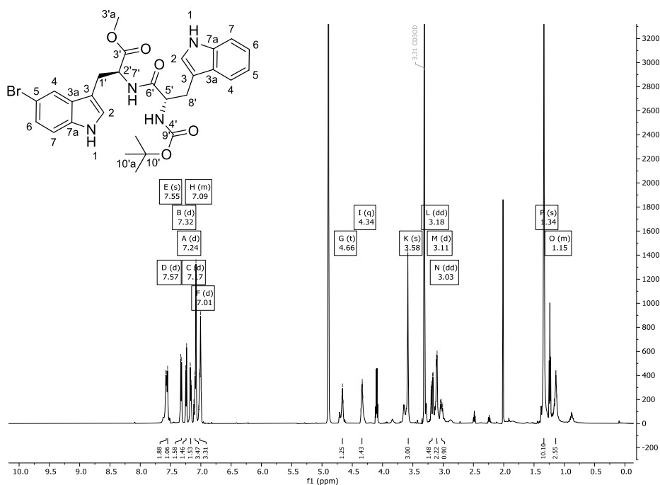
Abbildung 251: ^1\text{H} -NMR-Spektrum (600 MHz) von Verbindung 286 in \text{CD}_3\text{OD} .
