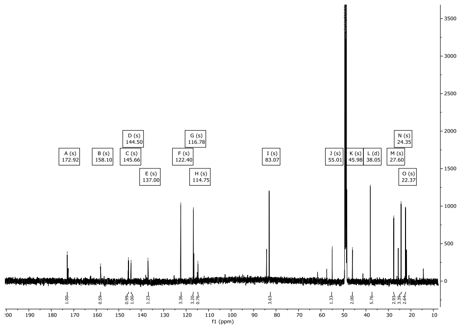
Abbildung 234: ^{13}\text{C} -NMR-Spektrum (151 MHz) von Verbindung 196 in \text{CD}_3\text{OD} .
