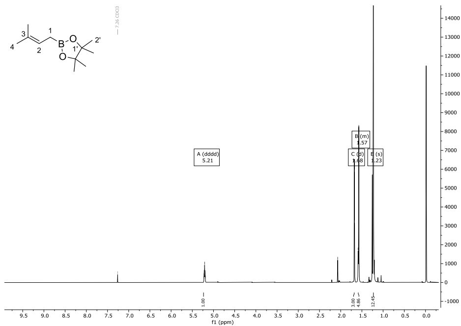
Abbildung 303: ^1\text{H} -NMR-Spektrum (600 MHz) von Verbindung 49 in \text{CDCl}_3 .
