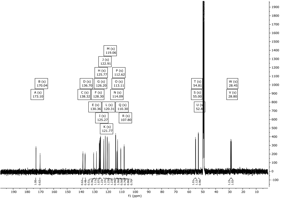
Abbildung 254: 13 C-NMR-Spektrum (151 MHz) von Verbindung 287 in CD 3 OD.
