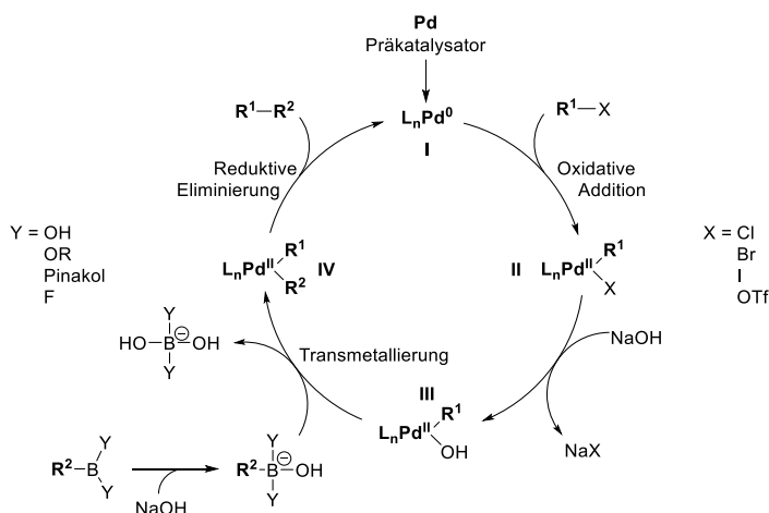
Schema 4: Katalysezyklus einer allgemeinen Suzuki-Miyaura-Kreuzkupplung mithilfe eines Palladium-Katalysators und Natriumhydroxid als Base. [85, 86]
