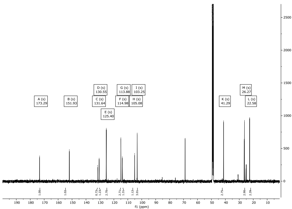
Abbildung 216: 13 C-NMR-Spektrum (151 MHz) von Verbindung 177 in CD 3 OD.
