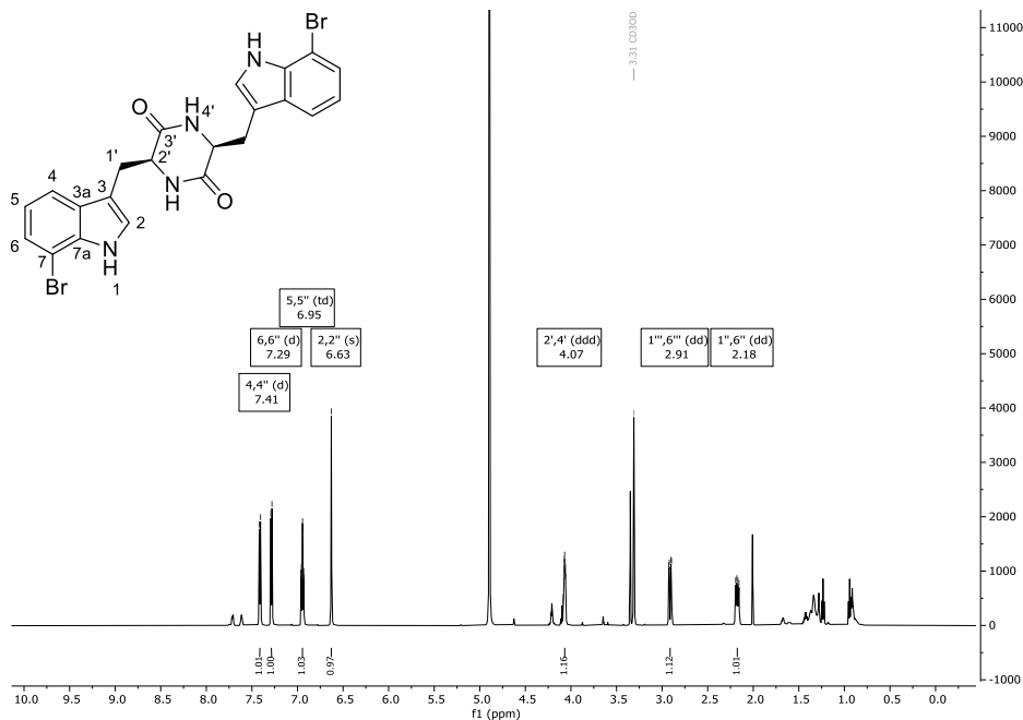
Abbildung 281: ^1\text{H} -NMR-Spektrum (600 MHz) von Verbindung 319 in \text{CD}_3\text{OD} .
