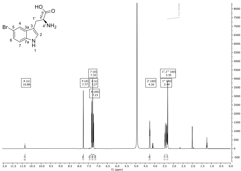
Abbildung 134: ^1\text{H} -NMR-Spektrum (600 MHz) von Verbindung 268 in \text{CD}_3\text{OD} .
