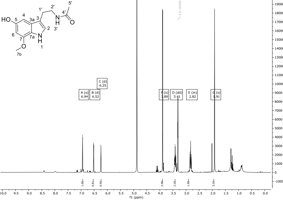
Abbildung 217: ^1\text{H} -NMR-Spektrum (600 MHz) von Verbindung 194 in \text{CD}_3\text{OD} .
