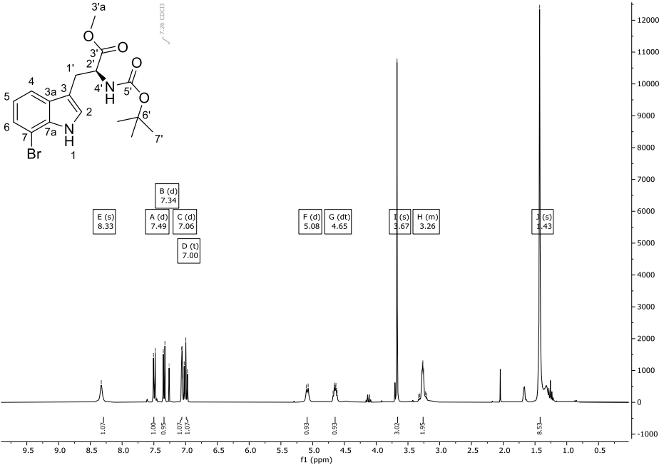
Abbildung 104: ^1\text{H} -NMR-Spektrum (300 MHz) von Verbindung 104 in \text{CDCl}_3 .
