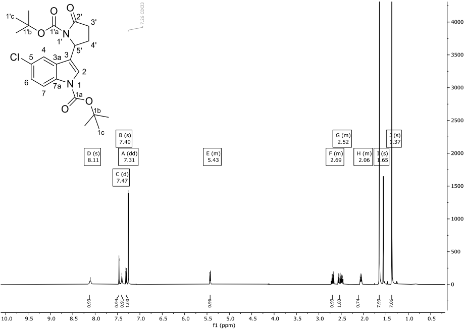
Abbildung 160: ^1\text{H} -NMR-Spektrum (600 MHz) von Verbindung 89 in \text{CDCl}_3 .
