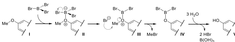
Schema 34: Vereinfachter, unimolekularer Mechanismus der \text{BBr}_3 -Entschützung eines aromatischen Methylethers. [196]
