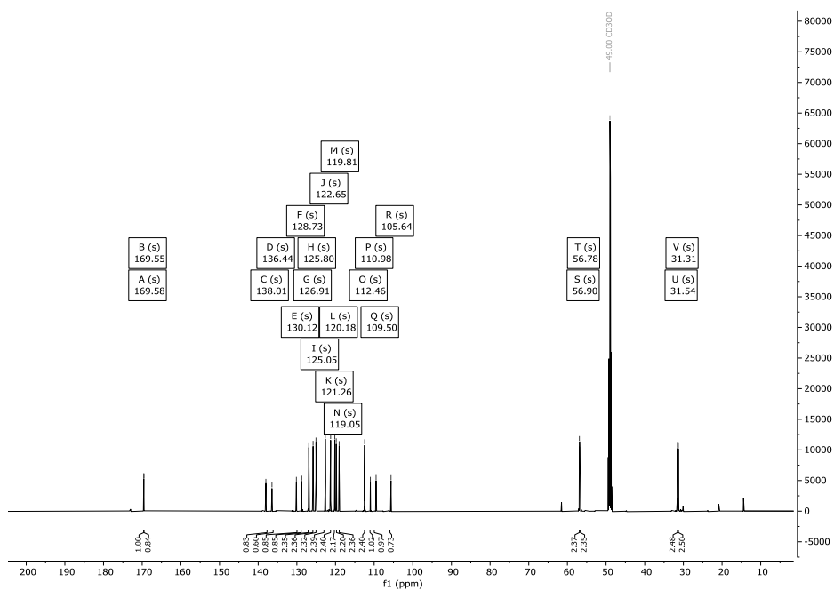
Abbildung 268: ^{13}\text{C} -NMR-Spektrum (151 MHz) von Verbindung 318 in \text{CD}_3\text{OD} .
