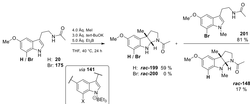
Schema 38: Dearomatisierende Zyklisierung von Melatonin 20 und 7-Brommelatonin 175 mithilfe von Triethylborat nach You et al. [180] und Hashim et al. [181]
