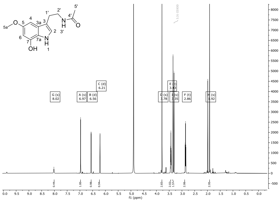
Abbildung 207: 1 H-NMR-Spektrum (600 MHz) von Verbindung 182 in CD 3 OD.
