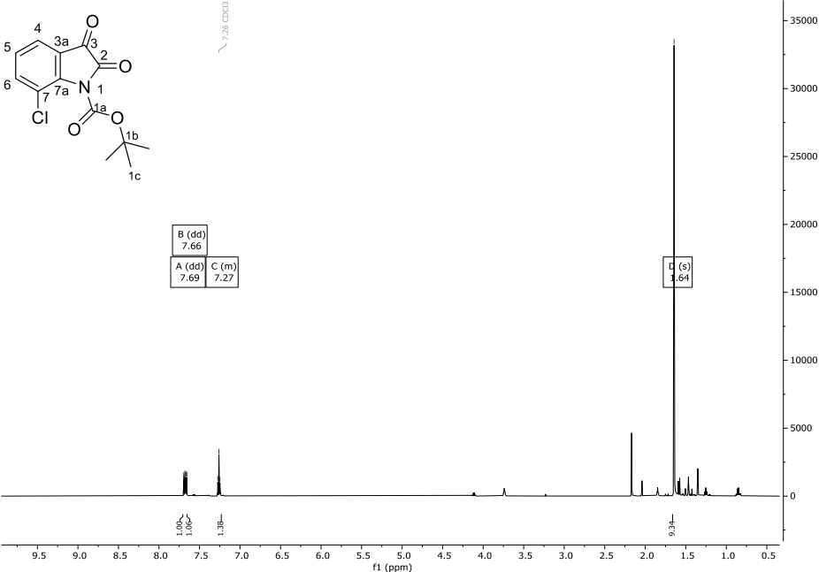
Abbildung 164: ^1\text{H} -NMR-Spektrum (600 MHz) von Verbindung 94 in \text{CDCl}_3 .
