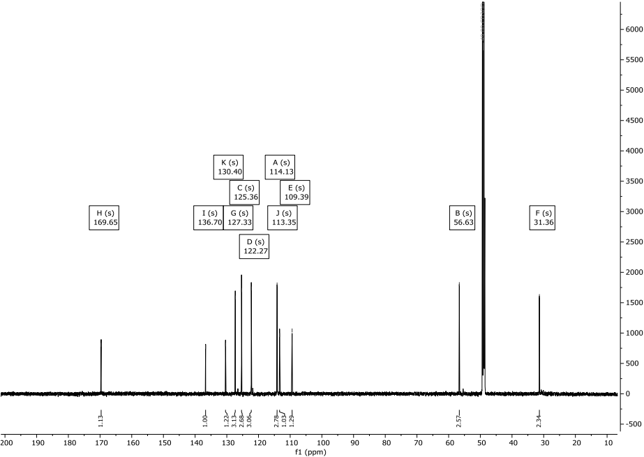
Abbildung 278: 13 C-NMR-Spektrum (151 MHz) von Verbindung 315 in CD 3 OD.
