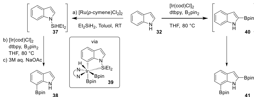
Schema 1: Hydrosilyl-dirigierte Borylierung in 7-Position im Vergleich zu einer ungerichteten Borylierung, welche zunächst in 2-Position und dann in 7-Position erfolgt, nach Hartwig et al. [83]
