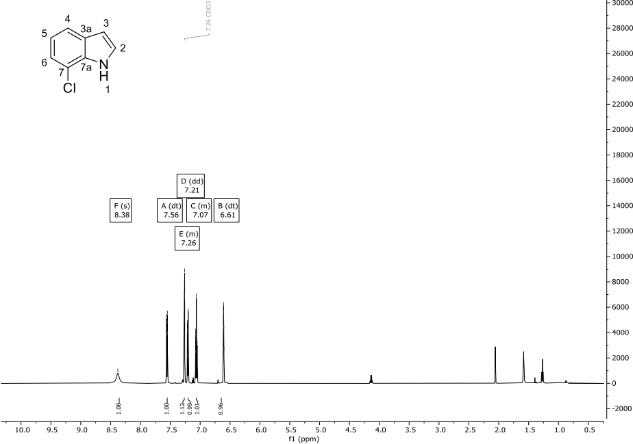
Abbildung 144: 1 H-NMR-Spektrum (300 MHz) von Verbindung 45 in CDCl 3 .
