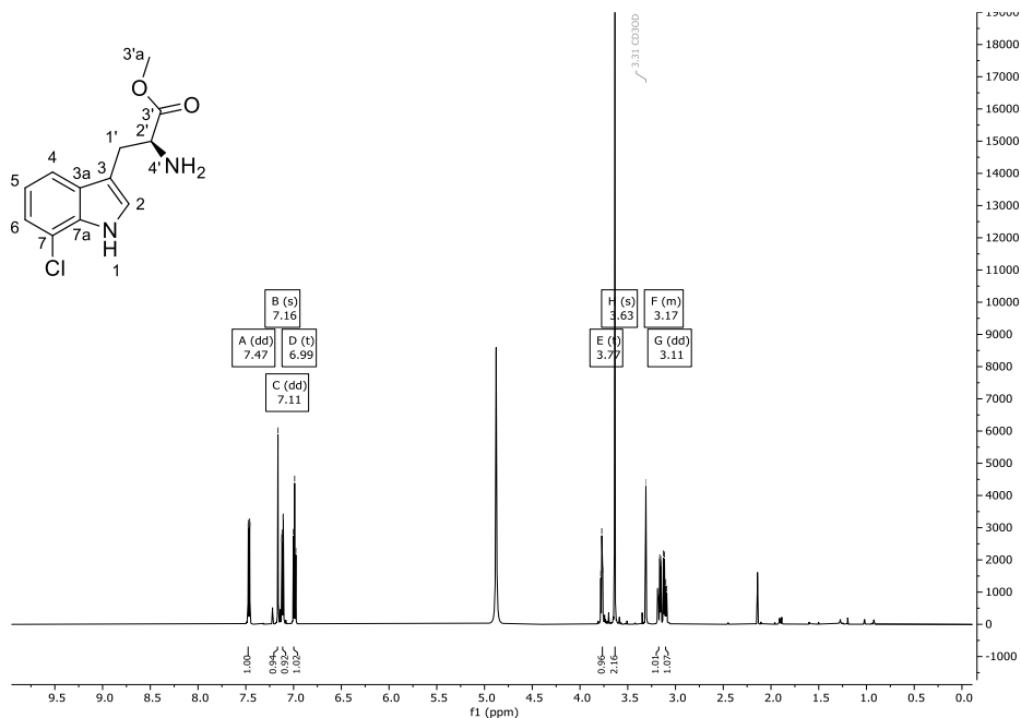
Abbildung 124: 1 H-NMR-Spektrum (600 MHz) von Verbindung 115 in CD 3 OD.
