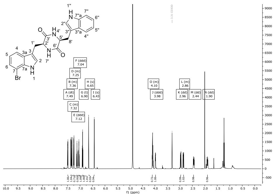
Abbildung 267: ^1\text{H} -NMR-Spektrum (600 MHz) von Verbindung 318 in \text{CD}_3\text{OD} .
