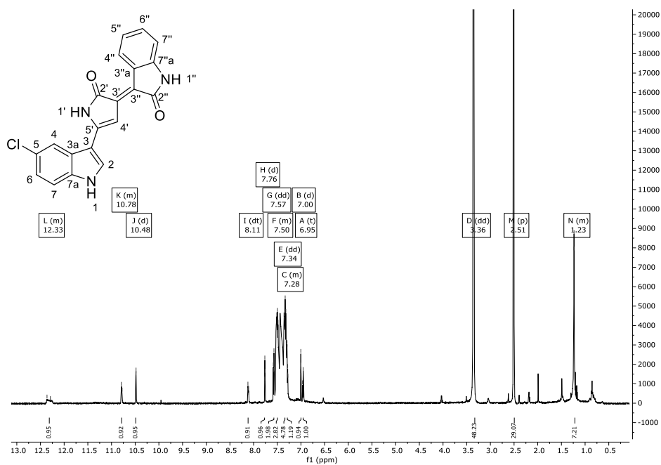
Abbildung 177: ^1\text{H} -NMR-Spektrum (600 MHz) der blauen Fraktion von Verbindung 95 in \text{d}_6\text{-DMSO} .
