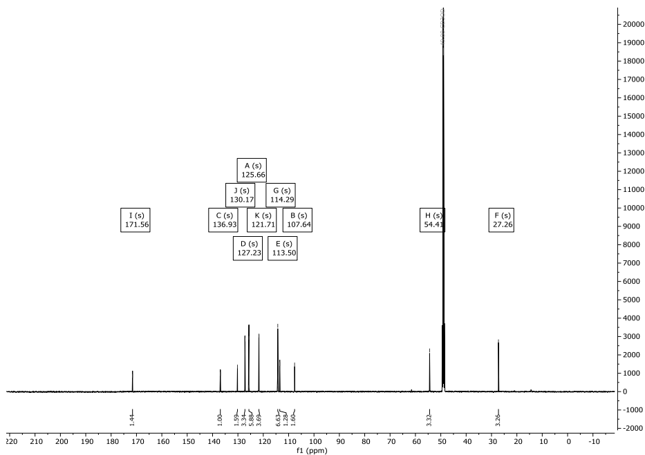
Abbildung 135: ^{13}\text{C} -NMR-Spektrum (151 MHz) von Verbindung 268 in \text{CD}_3\text{OD} .
