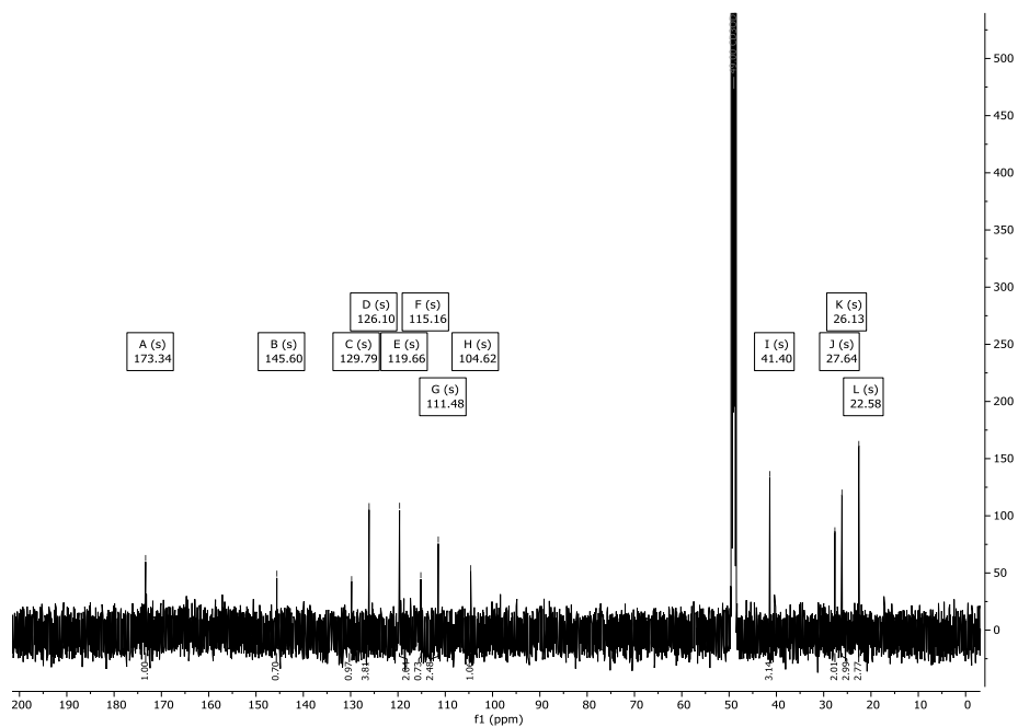
Abbildung 224: 13 C-NMR-Spektrum (151 MHz) von Verbindung 179 in CD 3 OD.
