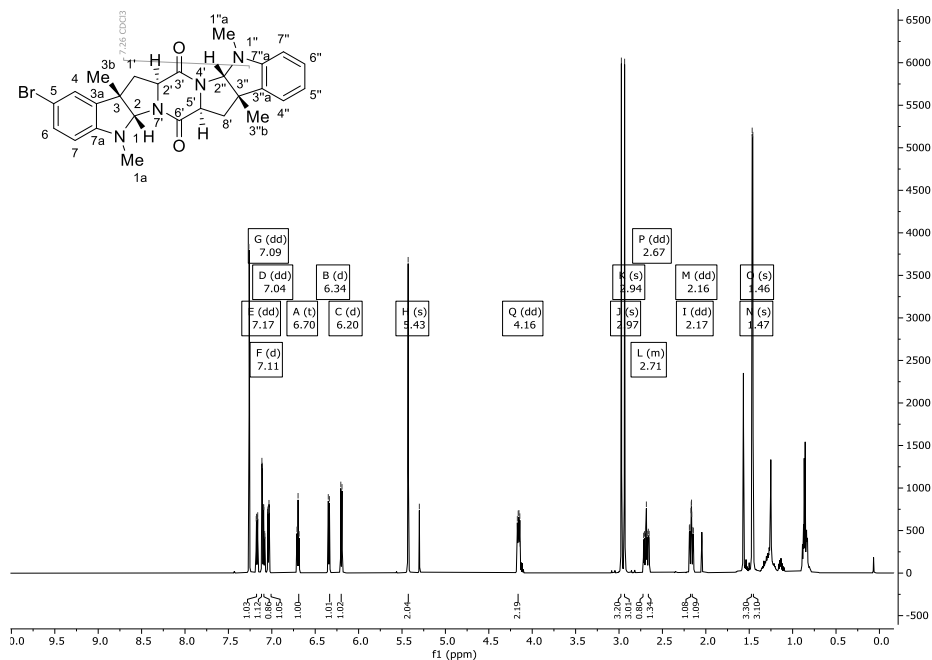
Abbildung 320: ^1\text{H} -NMR-Spektrum (600 MHz) von Verbindung 293 in \text{CDCl}_3 .
