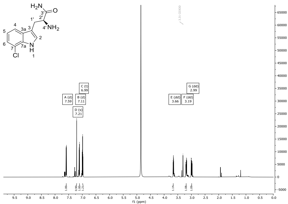
Abbildung 126: ^1\text{H-NMR} -Spektrum (600 MHz) von Verbindung 116 in \text{CD}_3\text{OD} .
