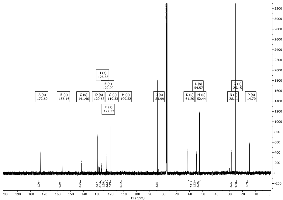
Abbildung 99: 13 C-NMR-Spektrum (151 MHz) von Verbindung 111 in CDCl 3 .
