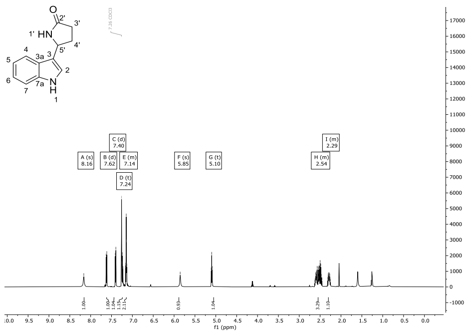
Abbildung 150: ^1\text{H-NMR} -Spektrum (600 MHz) von Verbindung 68 in \text{CDCl}_3 .
