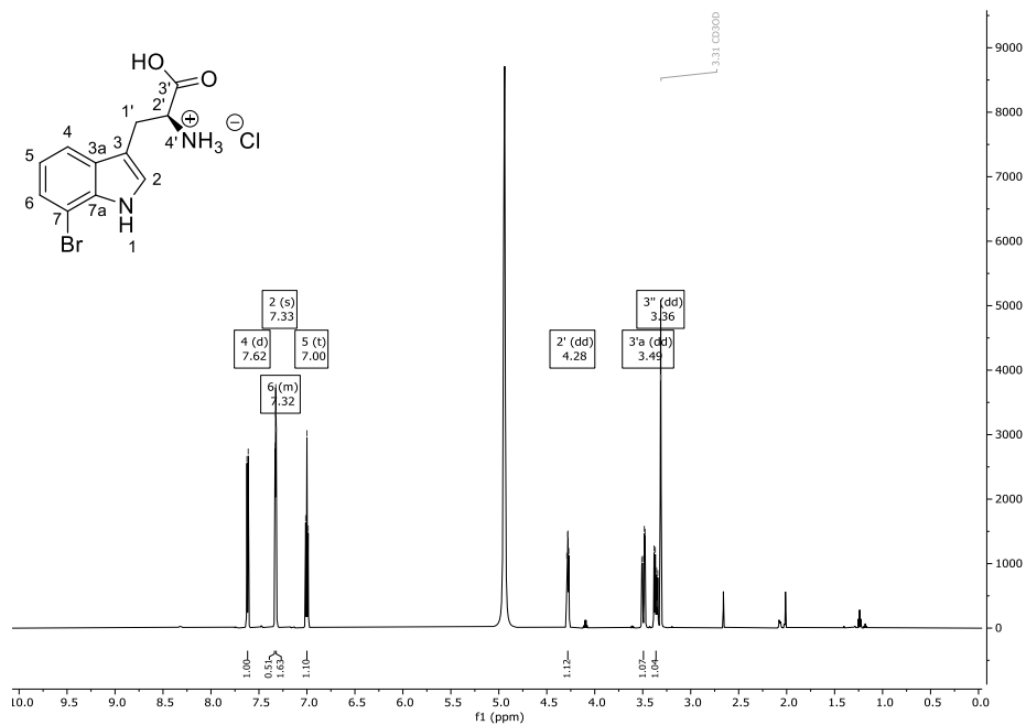
Abbildung 122: 1 H-NMR-Spektrum (600 MHz) von Verbindung 107-HCl in CD 3 OD.
