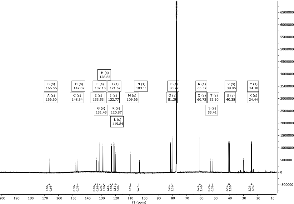
Abbildung 302: ^{13}\text{C} -NMR-Spektrum (226 MHz) von Verbindung 327 in \text{CDCl}_3 .
