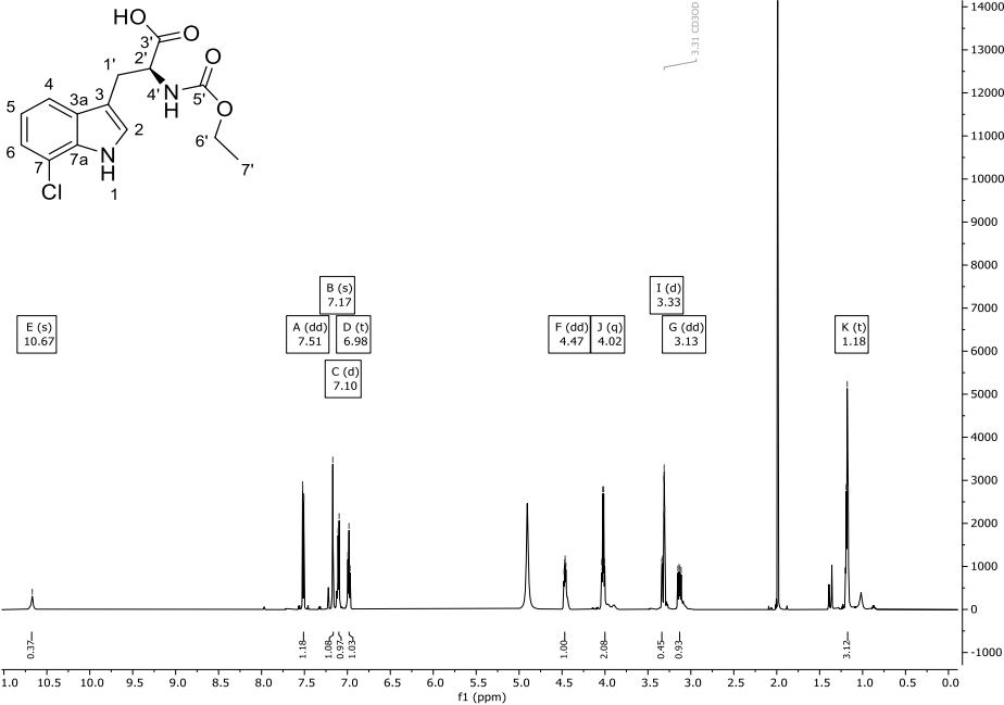
Abbildung 108: ^1\text{H} -NMR-Spektrum (600 MHz) von Verbindung 344 in \text{CD}_3\text{OD} .
