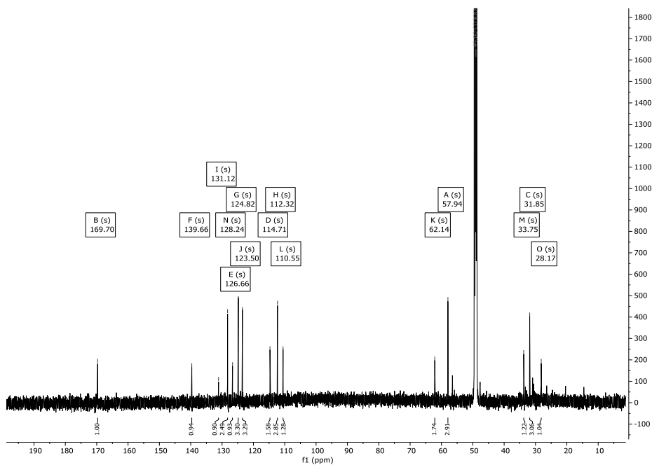
Abbildung 276: 13 C-NMR-Spektrum (151 MHz) von Verbindung 314 in CD 3 OD.
