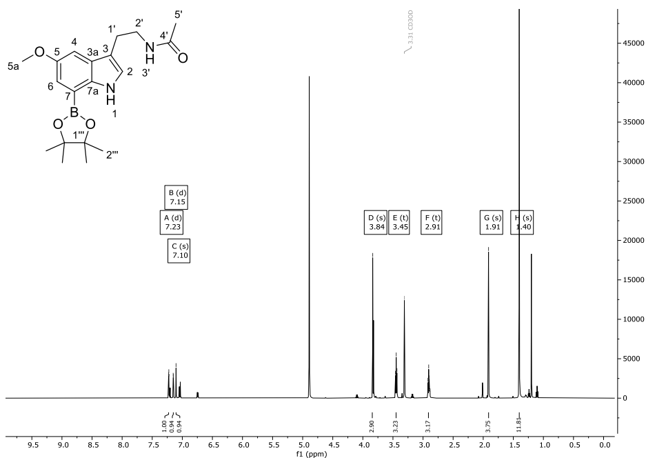
Abbildung 191: ^{13}\text{C} -NMR-Spektrum (151 MHz) von Verbindung 171 in \text{CD}_3\text{OD} .
