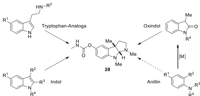
Schema 21: Mögliche Syntheserouten zum Physostigmin ( 28 ) ausgehend von funktionalisierten Indolen, Oxindolen, Tryptophanen und Anilinen.
