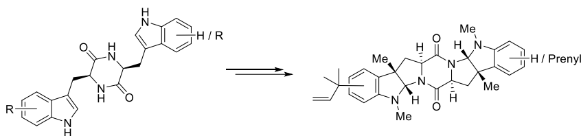
Schema 60: Schematische Darstellung der anvisierten Lansai-B-Derivate, welche über die neu-etablierte Totalsynthese mittels Methyltransferase SgmT erreicht werden können.
