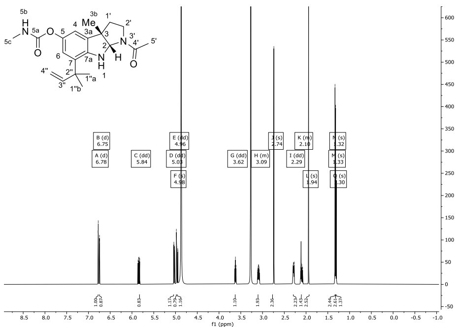
Abbildung 243: Synthetisches 1 H-NMR-Spektrum (700 MHz) des prädominanten Rotamers von Verbindung 203 in CD 3 OD.
