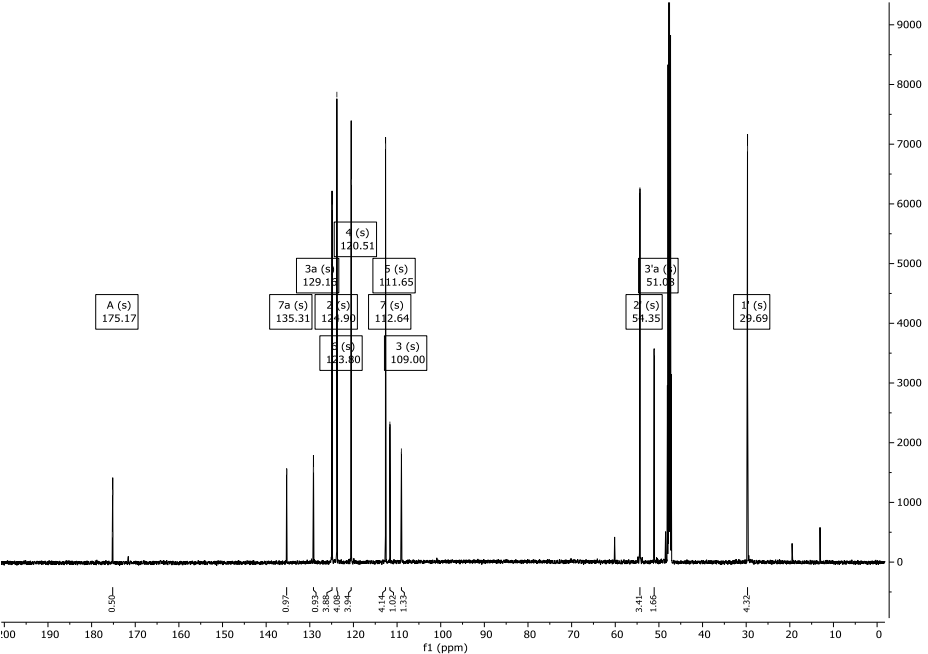
Abbildung 250: 13 C-NMR-Spektrum (151 MHz) von Verbindung 270 in CD 3 OD.
