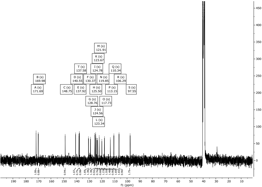
Abbildung 183: ^{13}\text{C} -NMR-Spektrum (151 MHz) von Verbindung 97 in \text{d}_6\text{-DMSO} .
