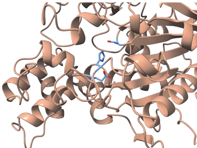
Abbildung 50: Kristallstruktur der AChE aus Electrophorus electricus (PDB: 1EEA) mit hervorgehobener katalytischer Triade (blau), bestehend aus S 200 , H 440 und E 327 . [207]
