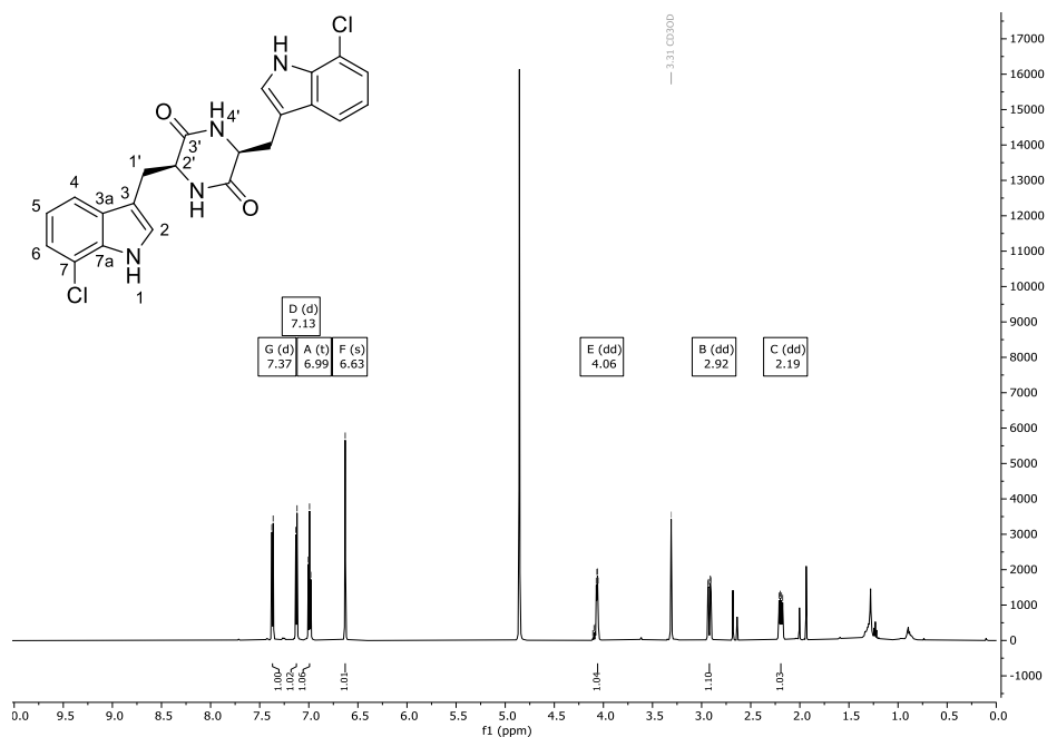
Abbildung 283: ^1\text{H} -NMR-Spektrum (600 MHz) von Verbindung 321 in \text{CD}_3\text{OD} .
