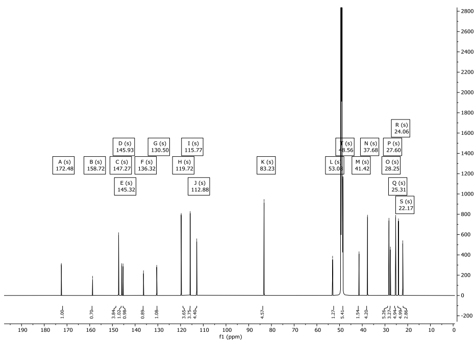
Abbildung 244: Synthetisches 13 C-NMR-Spektrum (176 MHz) des prädominanten Rotamers von Verbindung 203 in CD 3 OD.
