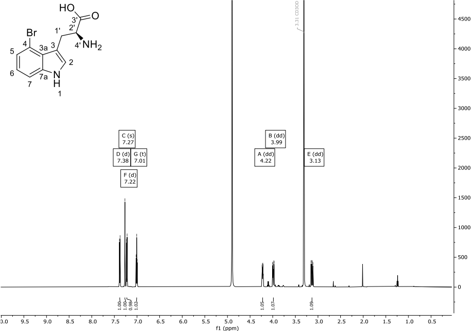
Abbildung 132: 1 H-NMR-Spektrum (600 MHz) von Verbindung 297 in CD 3 OD.
