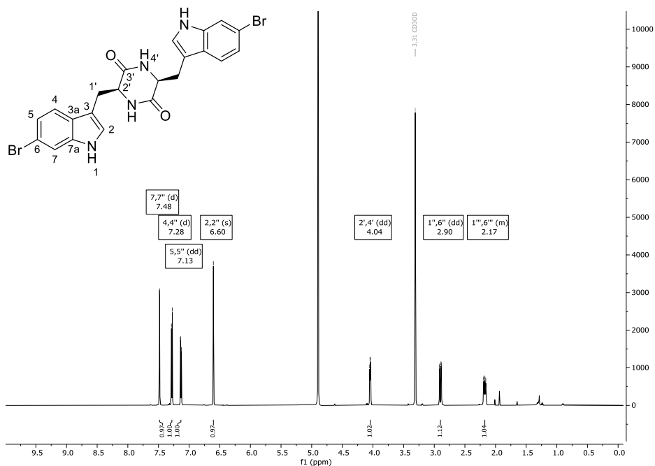
Abbildung 279: ^1\text{H} -NMR-Spektrum (600 MHz) von Verbindung 317 in \text{CD}_3\text{OD} .
