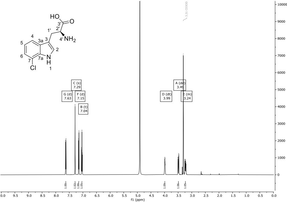
Abbildung 140: ^1\text{H} -NMR-Spektrum (600 MHz) von Verbindung 82 in \text{CD}_3\text{OD} .
