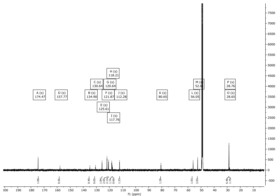
Abbildung 103: ^{13}\text{C} -NMR-Spektrum (151 MHz) von Verbindung 103 in \text{CD}_3\text{OD} .
