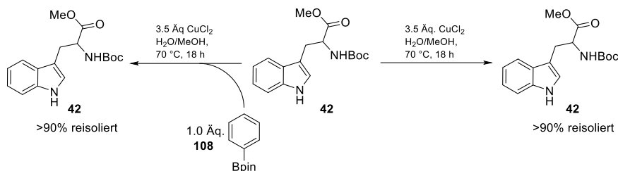
Schema 14: Untersuchung der Stabilität des Boc-geschützten Tryptophanmethylesters 42 unter Chlorierungsbedingungen unter Ausschluss/Zugabe eines Boronsäureesters.
