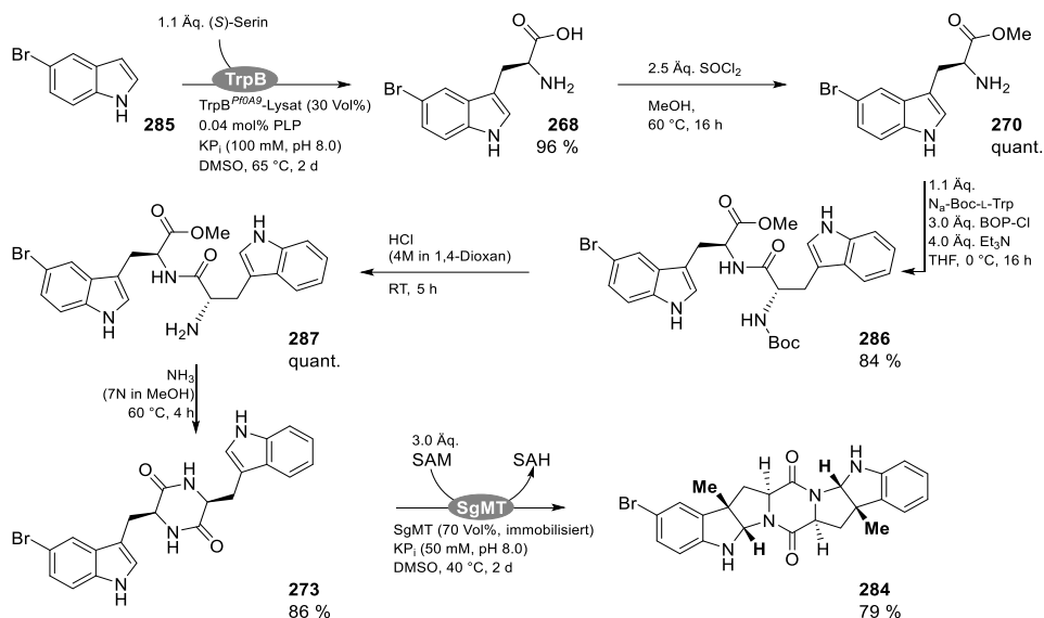
Schema 55: Enantiomerenreine Synthese von HHP 284 , ausgehend von 5-Bromindol 285 mithilfe der Tryptophan-Synthase Pj0A9 und der Methyltransferase SgMT.
