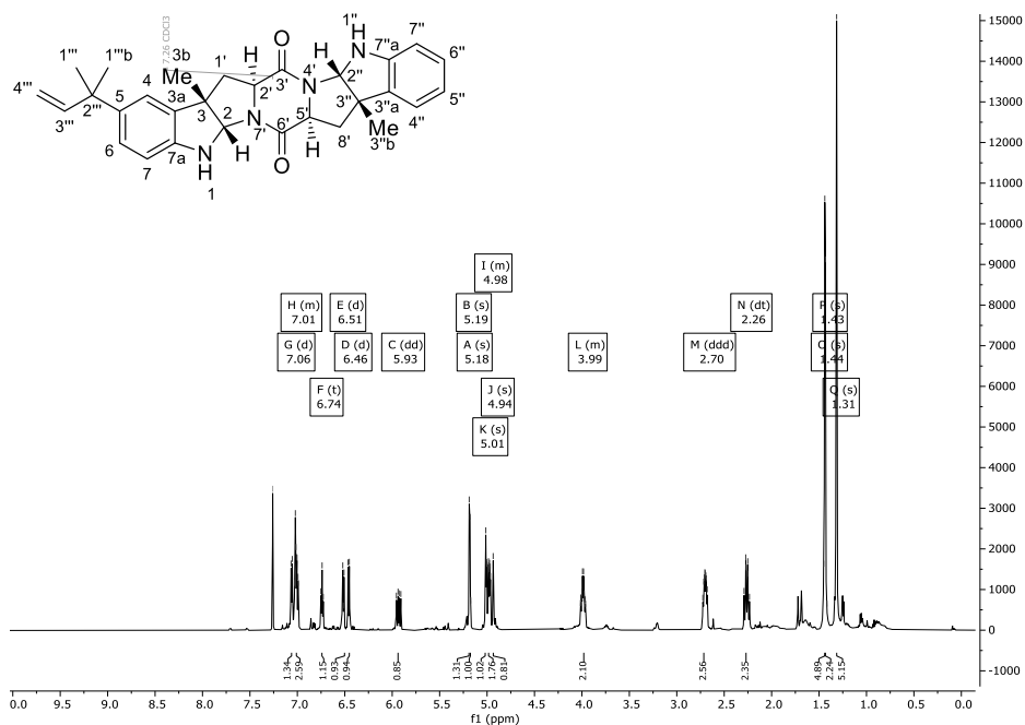
Abbildung 310: ^1\text{H} -NMR-Spektrum (600 MHz) von Verbindung 281 in \text{CDCl}_3 .
