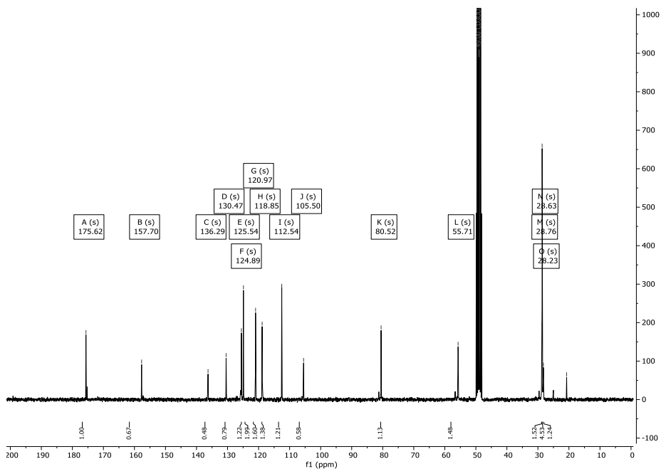
Abbildung 119: ^{13}\text{C} -NMR-Spektrum (151 MHz) von Verbindung 106 in \text{CD}_3\text{OD} .
