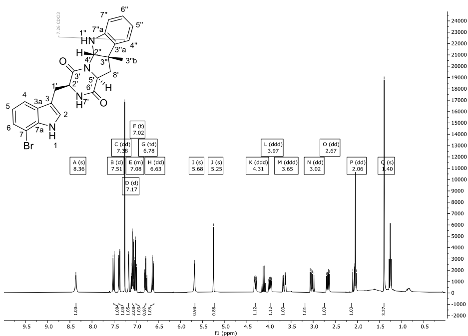
Abbildung 299: ^1\text{H} -NMR-Spektrum (900 MHz) von Verbindung 332 in \text{CDCl}_3 .
