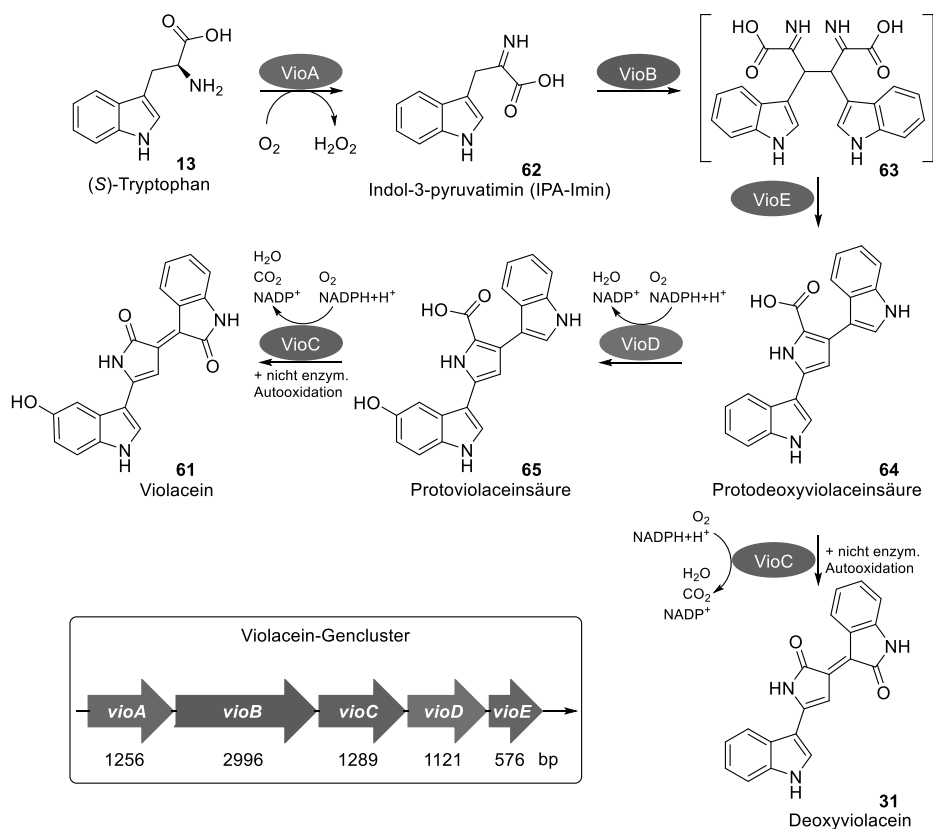
Schema 8: Aus C. violaceum identifizierter Gencluster und die daraus entwickelte Biosyntheseroute zum Violacein ( 61 ) und Deoxyviolacein ( 31 ) von August et al. und Balibar. [126, 128]
