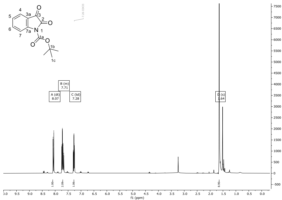
Abbildung 162: ^1\text{H} -NMR-Spektrum (600 MHz) von Verbindung 72 in \text{CDCl}_3 .
