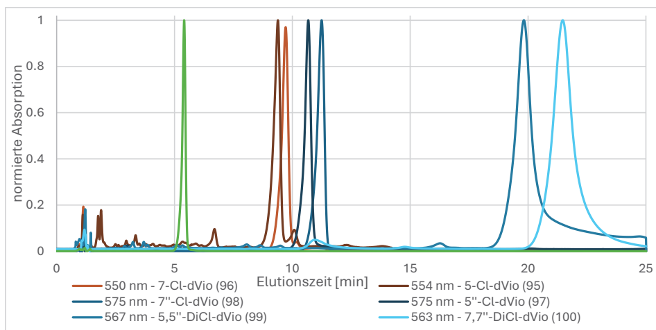
Abbildung 20: Überlagertes Chromatogramm aller sechs verschiedenen dVio-Derivate und des natürlichen dVio bei gleichbleibender HPLC-Methode (Isaspher C18-Säule mit Wasser/Acetonitril: 55/45). Aufgetragen ist die Absorption (normiert auf den höchsten Absorptionswert) bei der maximalen Absorptionswellenlänge gegen die Elutionszeit.
