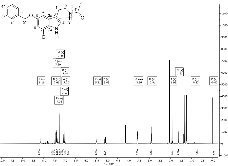
Abbildung 193: 1 H-NMR-Spektrum (600 MHz) von Verbindung 172 in CDCl 3 .
