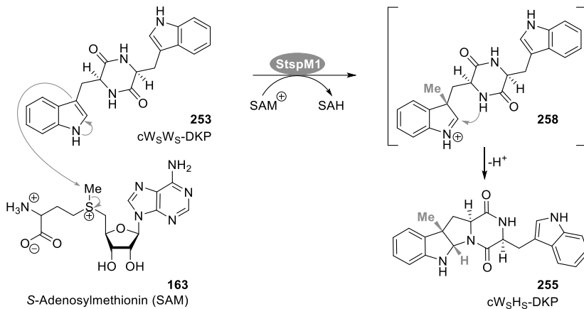
Schema 49: Katalysierte Reaktion der Methyltransferase StspM1 beschrieben von Zhu et al. [58]
