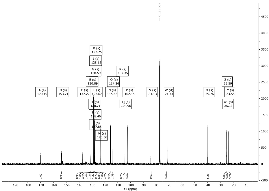
Abbildung 196: ^{13}\text{C} -NMR-Spektrum (151 MHz) von Verbindung 174 in \text{CDCl}_3 .
