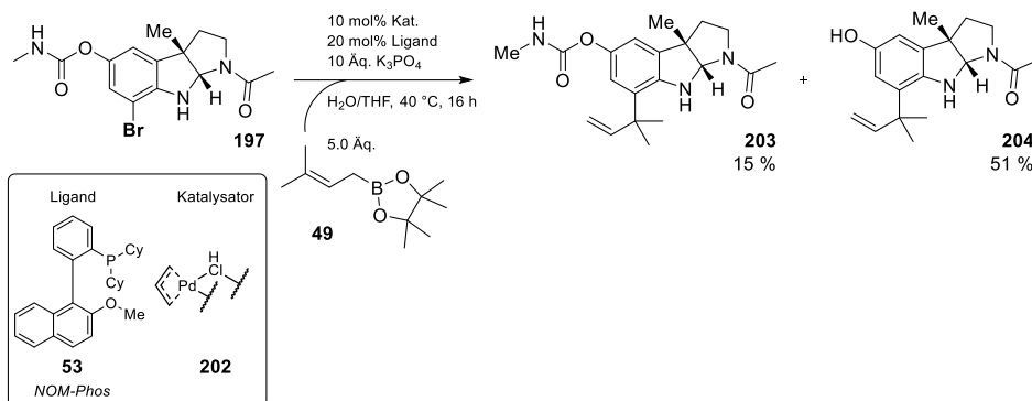
Schema 39: Suzuki-Kreuzkupplung von 7-Brom-HHP 197 zur entsprechenden Prenylverbindung 203 nach Buchwald. [89]
