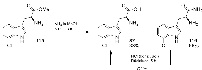
Schema 16: Hydrolyse des Esters 115 mithilfe von Ammoniak in Methanol zum Amid 116 und nachfolgend durchgeführte Umwandlung zur Carbonsäure 82 .
