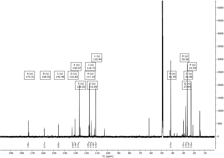
Abbildung 222: 13 C-NMR-Spektrum (151 MHz) von Verbindung 178 in CD 3 OD.
