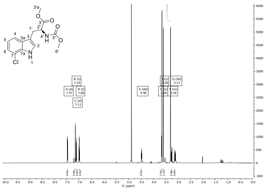
Abbildung 110: ^1\text{H} -NMR-Spektrum (600 MHz) von Verbindung 114 in \text{CD}_3\text{OD} .
