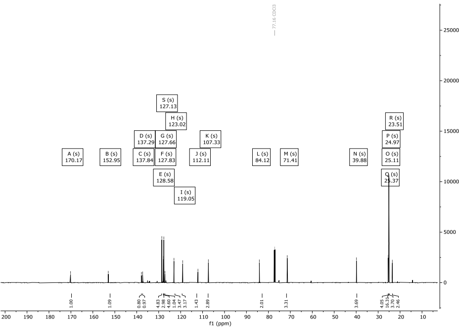
Abbildung 190: ^{13}\text{C} -NMR-Spektrum (151 MHz) von Verbindung 170 in \text{CDCl}_3 .
