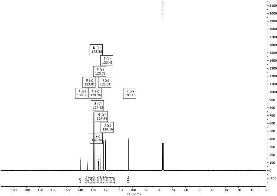
Abbildung 149: ^{13}\text{C} -NMR-Spektrum (76 MHz) von Verbindung 120 in \text{CDCl}_3 .
