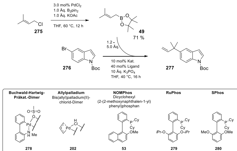
Schema 53: Synthese von Prenyl-Boronsäureester 49 und anschließendes screening von Katalysatoren und Liganden am Modellsubstrat 5-Bromindol 276 gemäß den Bedingungen von Reisman et al. [219] und Buchwald et al. [89]
