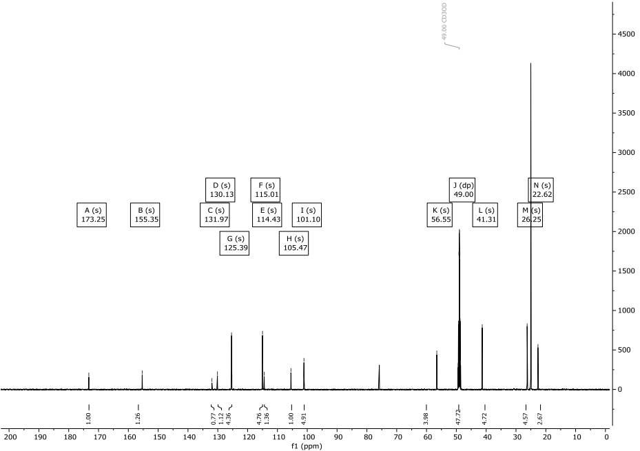
Abbildung 206: 13 C-NMR-Spektrum (600 MHz) von Verbindung 175 in CD 3 OD.
