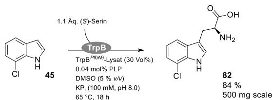
Schema 18: Chemoenzymatische Synthese von (S)-7-Chlortryptophan ( 82 ) mithilfe der Tryptophan-Synthase TrpB ProA9 . [103]
