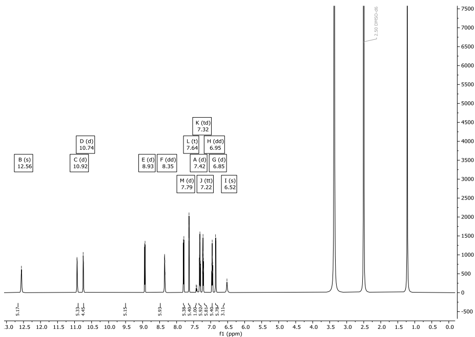
Abbildung 175: Synthetisches 1 H-NMR-Spektrum (600 MHz) der violetten Fraktion von Verbindung 96 in d 6 -DMSO.
