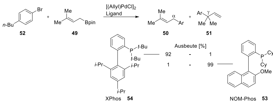
Schema 6: Reaktionsschema der ligandenkontrollierten, regiodivergenten Suzuki-Miyaura-Kreuzkupplungen nach Yang und Buchwald. [89]
