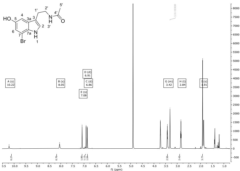
Abbildung 215: 1 H-NMR-Spektrum (600 MHz) von Verbindung 177 in CD 3 OD.
