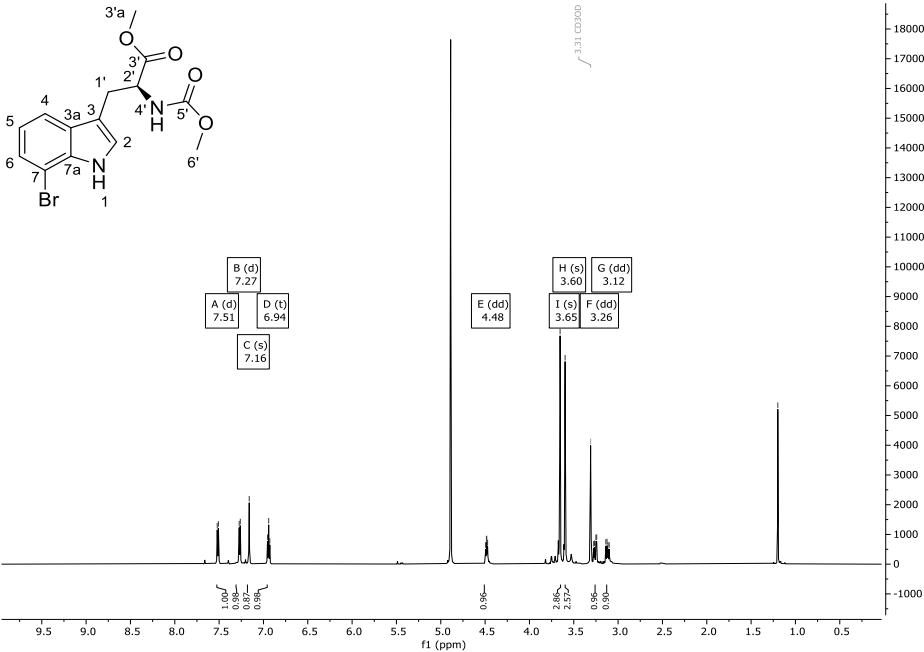
Abbildung 112: 1 H-NMR-Spektrum (600 MHz) von Verbindung 118 in CD 3 OD.
