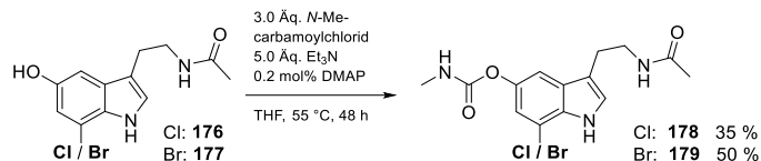
Schema 31: Carbamoylierung des chlorierten und bromierten Phenols 176 bzw. 177 .
