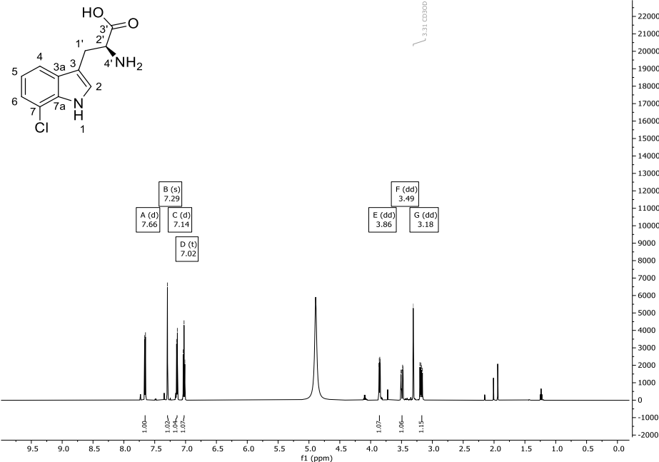
Abbildung 128: ^1\text{H} -NMR-Spektrum (600 MHz) von Verbindung 82 in \text{CD}_3\text{OD} .
