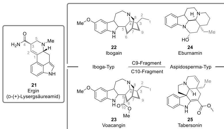
Abbildung 7: Chemische Struktur verschiedener isoprenoider Indolalkaloide. Das Terpengerüst ist grau markiert und nummeriert.
