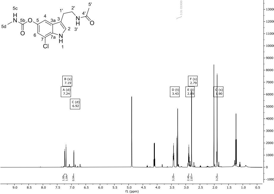
Abbildung 221: 1 H-NMR-Spektrum (600 MHz) von Verbindung 178 in CD 3 OD.
