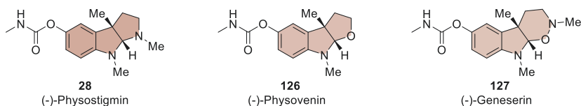
Abbildung 33: Chemische Struktur der aus der Kalabarbohne isolierten Indolalkaloide.
