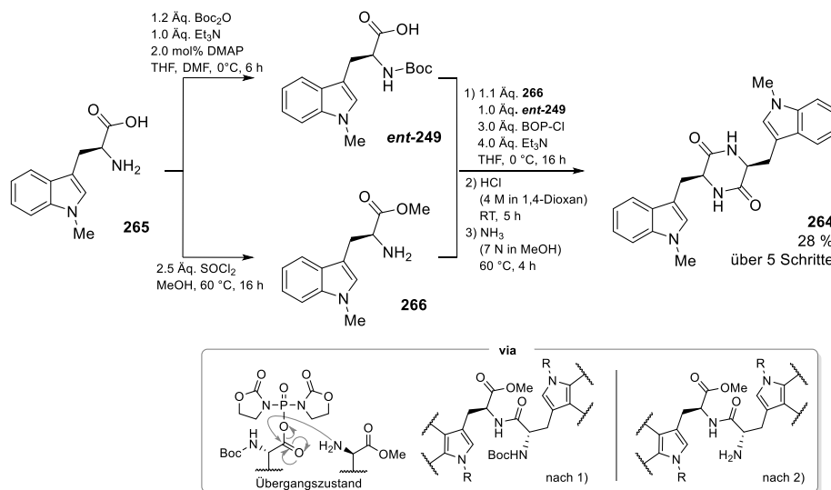
Schema 51: Synthese von N -Methyl-DKP 264 ausgehend von ( S )- N -Methyltryptophan 265 über eine Veresterung, Boc-Schätzung, Peptidknüpfung und anschließende Entschätzung der verwendeten PGs.
