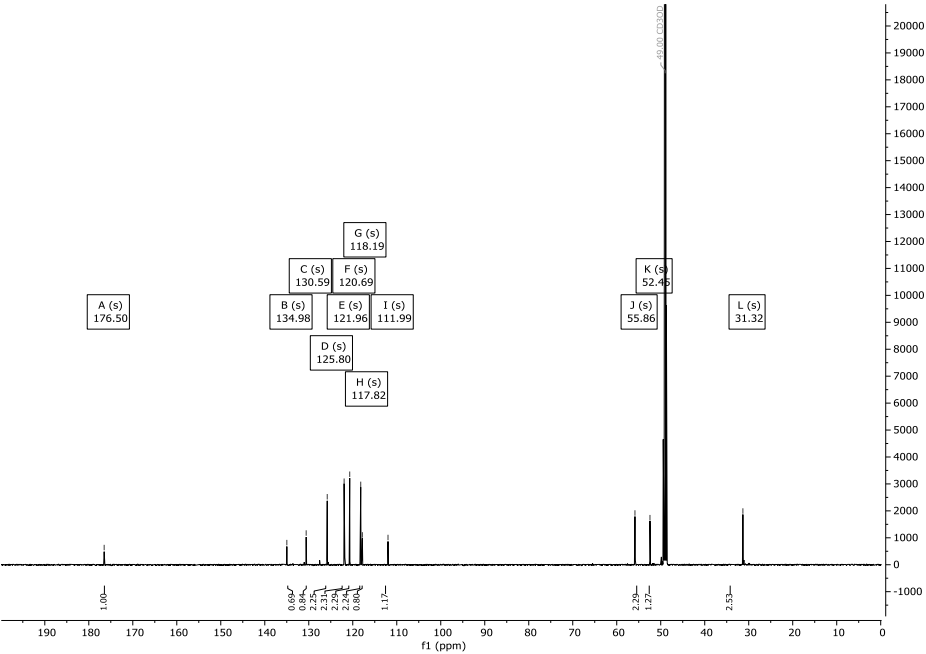
Abbildung 125: 13 C-NMR-Spektrum (600 MHz) von Verbindung 115 in CD 3 OD.
