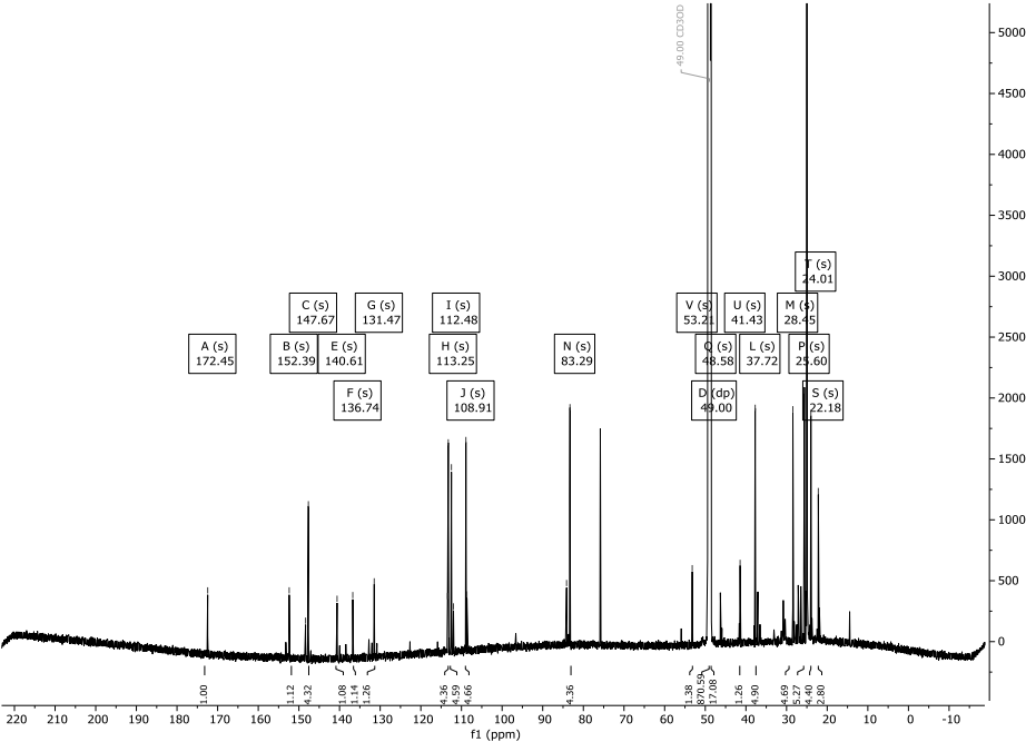
Abbildung 246: ^{13}\text{C} -NMR-Spektrum (176 MHz) von Verbindung 204 in \text{CD}_3\text{OD} .
