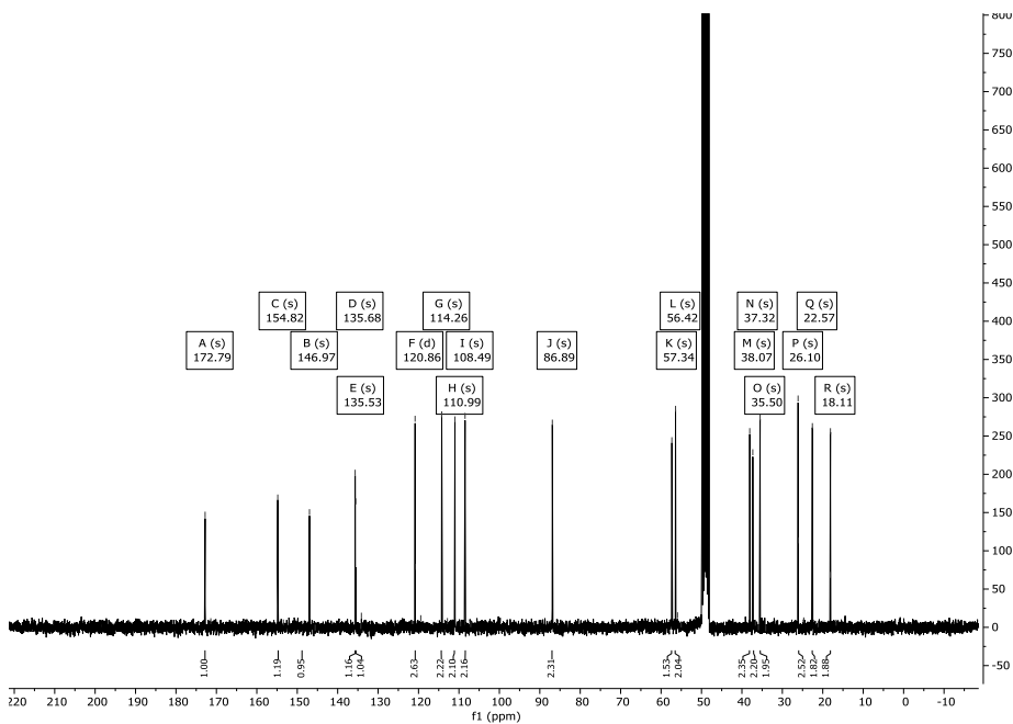
Abbildung 315: ^{13}\text{C} -NMR-Spektrum (76 MHz) von Verbindung 290 in \text{CD}_3\text{OD} .
