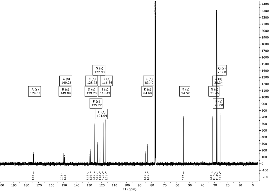
Abbildung 161: ^{13}\text{C} -NMR-Spektrum (151 MHz) von Verbindung 89 in \text{CDCl}_3 .
