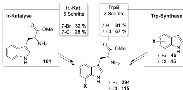
Schema 63: Vergleich der zwei Methoden zur Synthese des 7-bromierten und 7-chlorierten Tryptophanmethylesters 115 bzw. 294 über die Ir-katalysierte Tryptophan-Funktionalisierung oder die enzymatische Tryptophansynthese unter Angabe der Gesamtausbeuten.
