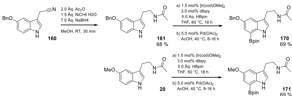
Schema 29: Reaktionsschema der CH-Aktivierung von Benzyloxy- und Methoxyindolamid 161 und 20 über 7-Borylierung.
