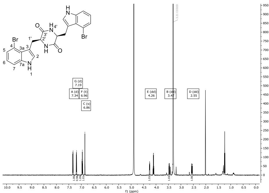
Abbildung 275: 1 H-NMR-Spektrum (600 MHz) von Verbindung 314 in CD 3 OD.
