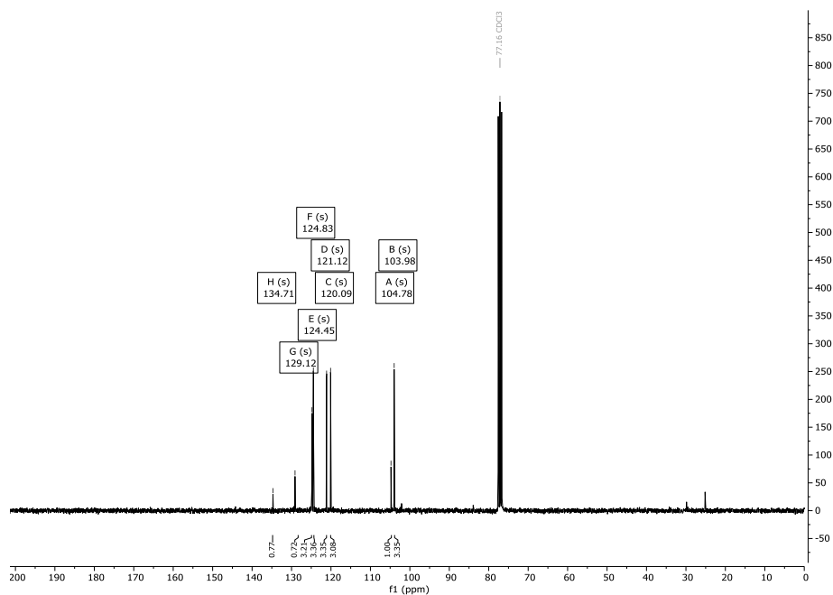
Abbildung 147: ^{13}\text{C} -NMR-Spektrum (76 MHz) von Verbindung 46 in \text{CDCl}_3 .
