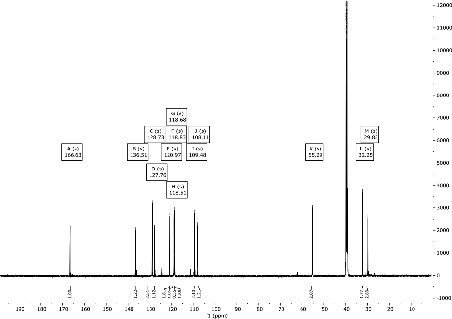
Abbildung 286: 13 C-NMR-Spektrum (151 MHz) von Verbindung 264 in d 6 -DMSO.
