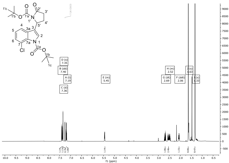
Abbildung 158: ^1\text{H} -NMR-Spektrum (600 MHz) von Verbindung 90 in \text{CDCl}_3 .
