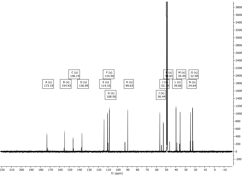
Abbildung 230: 13 C-NMR-Spektrum (151 MHz) von Verbindung rac -148 in CD 3 OD.
