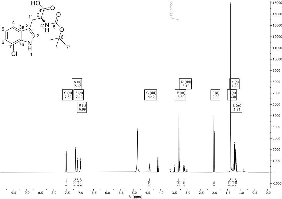
Abbildung 116: ^1\text{H} -NMR-Spektrum (600 MHz) von Verbindung 105 in \text{CD}_3\text{OD} .
