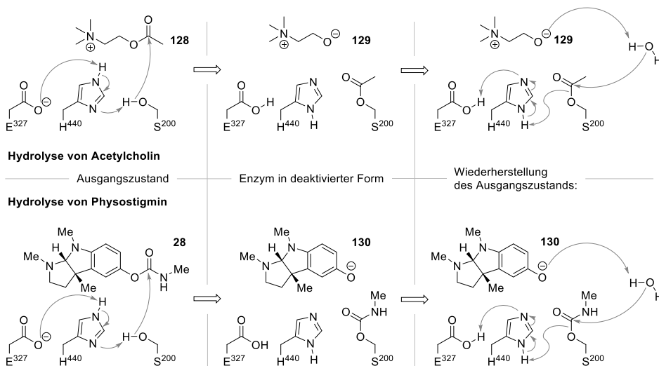
Schema 20: Katalyse-Mechanismus der hydrolytischen Spaltung von ACh bzw. Physostigmin (28) durch die AChE. [173] Die Regeneration des Ausgangszustands ist beim carbamoylierten Ser 200 (nach Umsetzung von Physostigmin) bedeutend langsamer als beim veresterten Ser 200 (nach Umsetzung von ACh).
