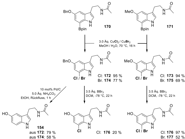
Schema 30: Reaktionsschema zur Funktionalisierung von Boronsäureester 170 bzw. 171 zum Chlorid/Bromid und anschließende Entschüttung der 5-Hydroxygruppen.
