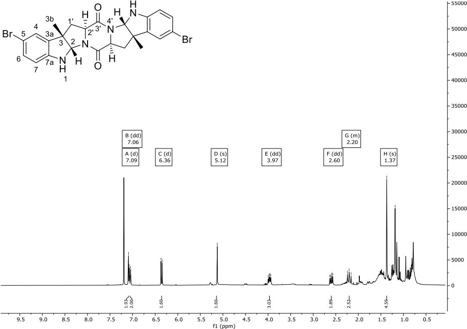
Abbildung 297: ^1\text{H} -NMR-Spektrum (300 MHz) von Verbindung 324 in \text{CDCl}_3 .
