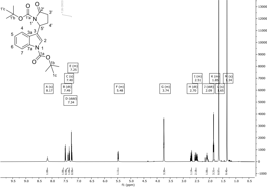
Abbildung 156: ^1\text{H} -NMR-Spektrum (600 MHz) von Verbindung 70 in \text{CDCl}_3 .
