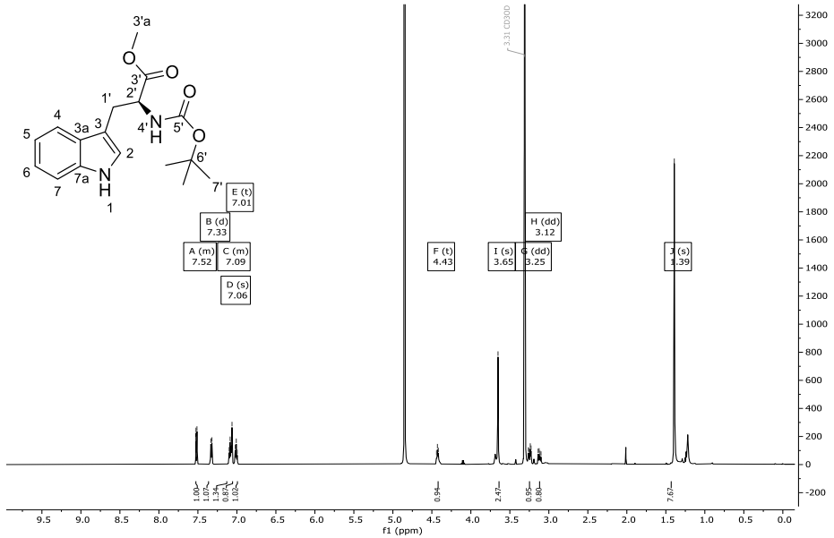
Abbildung 90: 1 H-NMR-Spektrum (600 MHz) von Verbindung 42 in CD 3 OD.
