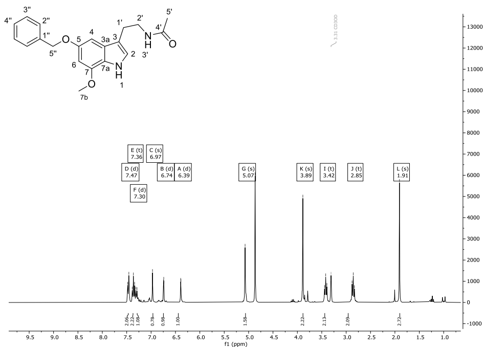
Abbildung 199: ^1\text{H} -NMR-Spektrum (600 MHz) von Verbindung 193 in \text{CD}_3\text{OD} .
