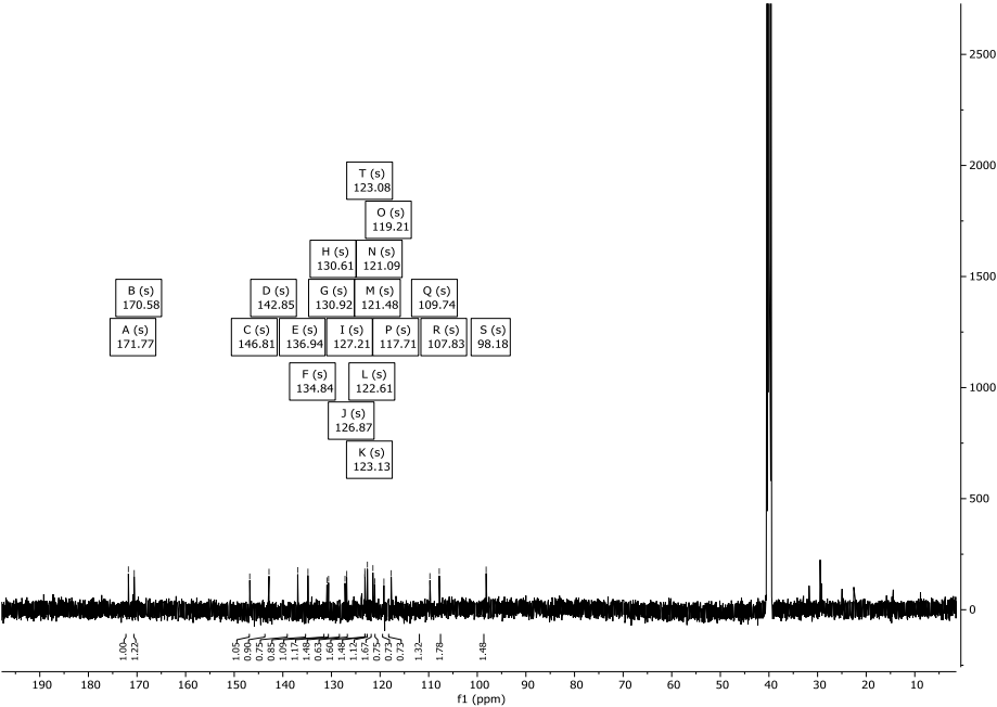
Abbildung 176: 13 C-NMR-Spektrum (151 MHz) der violetten Fraktion von Verbindung 96 in d 6 -DMSO.
