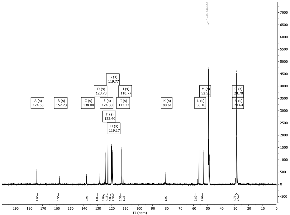
Abbildung 91: 13 C-NMR-Spektrum (151 MHz) von Verbindung 42 in CD 3 OD.
