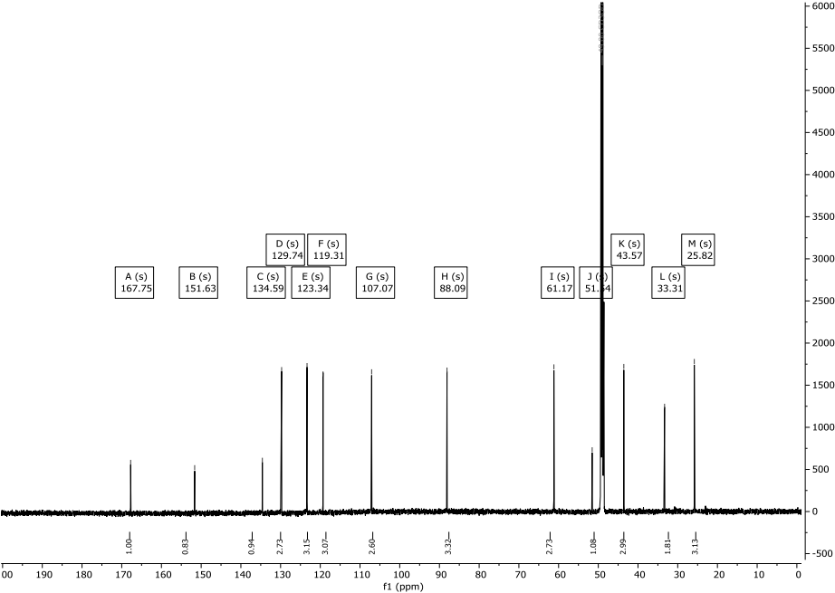
Abbildung 317: 13 C-NMR-Spektrum (151 MHz) von Verbindung 282 in CD 3 OD.
