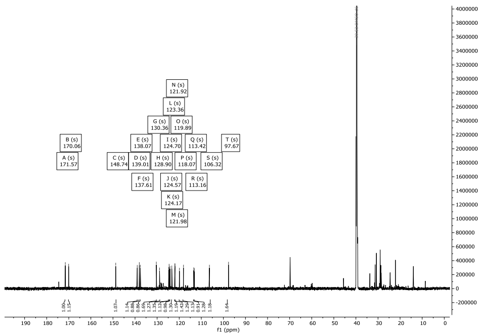
Abbildung 181: ^{13}\text{C} -NMR-Spektrum (151 MHz) der violetten Fraktion von Verbindung 98 in d_6 -DMSO.
