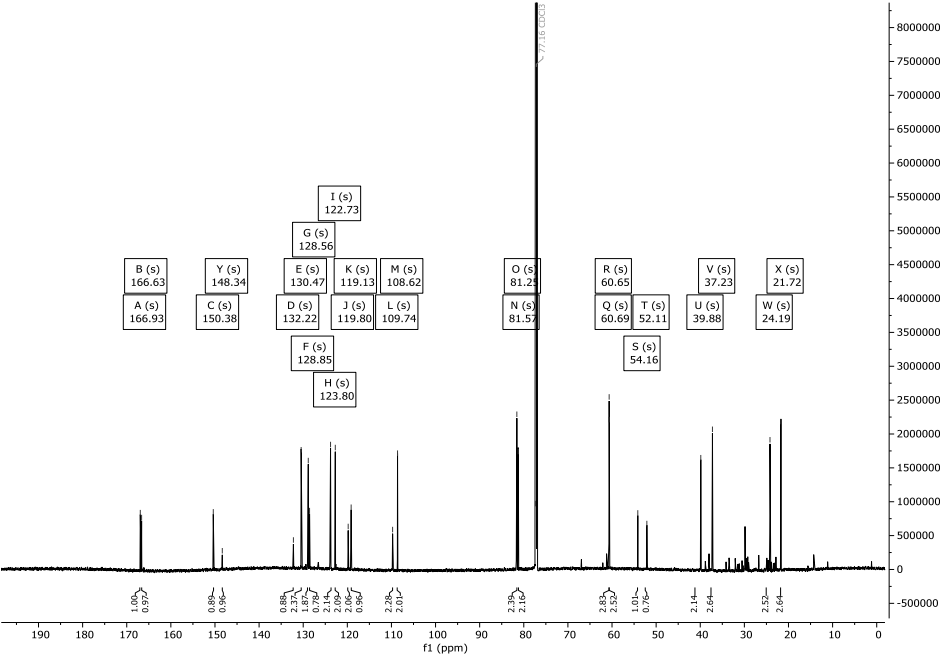
Abbildung 290: ^{13}\text{C} -NMR-Spektrum (226 MHz) von Verbindung 322 in \text{CDCl}_3 .
