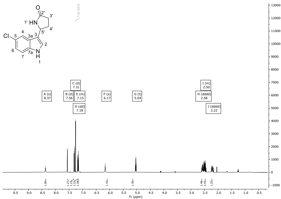
Abbildung 154: ^1\text{H} -NMR-Spektrum (600 MHz) von Verbindung 87 in \text{CDCl}_3 .
