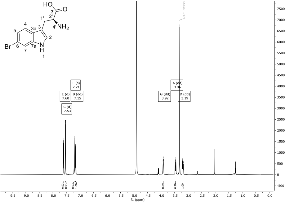
Abbildung 136: ^1\text{H} -NMR-Spektrum (600 MHz) von Verbindung 298 in \text{CD}_3\text{OD} .
