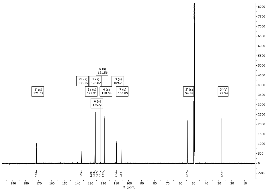
Abbildung 139: ^{13}\text{C} -NMR-Spektrum (151 MHz) von Verbindung 107 in \text{CD}_3\text{OD} .
