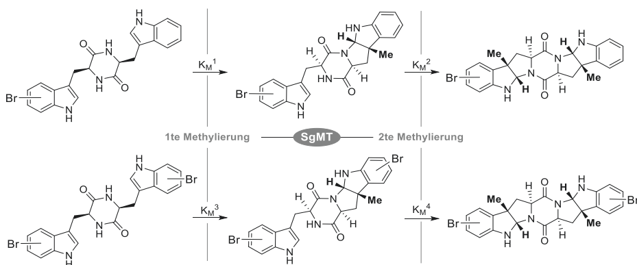
Schema 65: Einzelreaktionen der enzymatischen Methylierung. Für eine genaue Betrachtung der jeweiligen Reaktionskonstanten K_M^x müssten daher auch die einfach-methylierten Moleküle im Glo-Assay untersucht werden.
