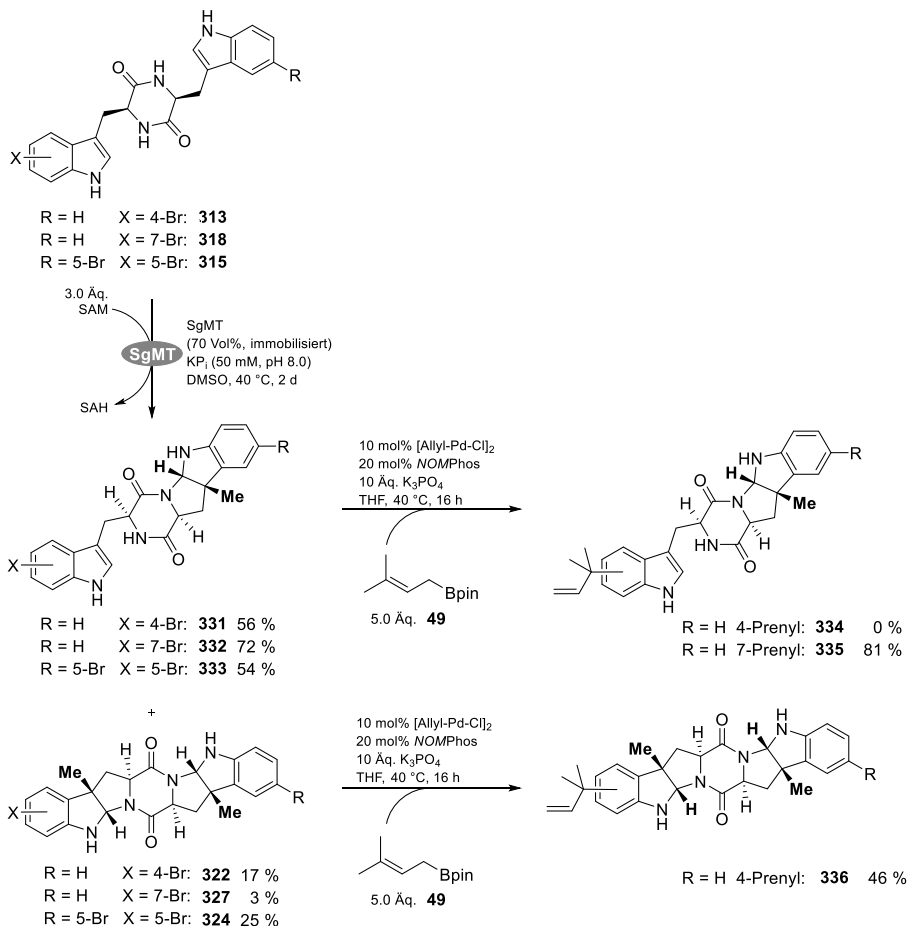
Schema 66: Enzymatische Methylierung und Palladium-katalysierte Prenylierung der 4-, 5- und 7-bromierten DKP-Derivate 313 , 315 und 318 . Die einfach- und doppelt-methylierten Produkte ( 331-333 , bzw. 322 , 324 und 327 ) wurden isoliert und einzeln für die Prenylierung eingesetzt.
