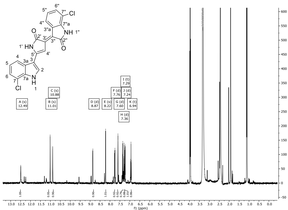
Abbildung 184: ^1\text{H} -NMR-Spektrum (600 MHz) von Verbindung 100 in d_6 -DMSO.
