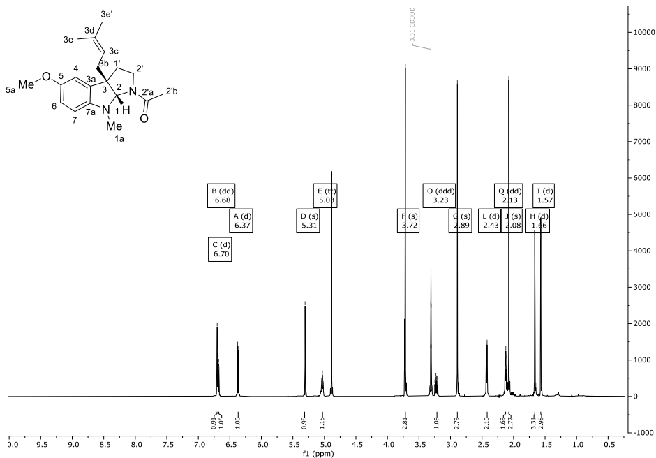
Abbildung 314: ^1\text{H} -NMR-Spektrum (600 MHz) von Verbindung 290 in \text{CD}_3\text{OD} .
