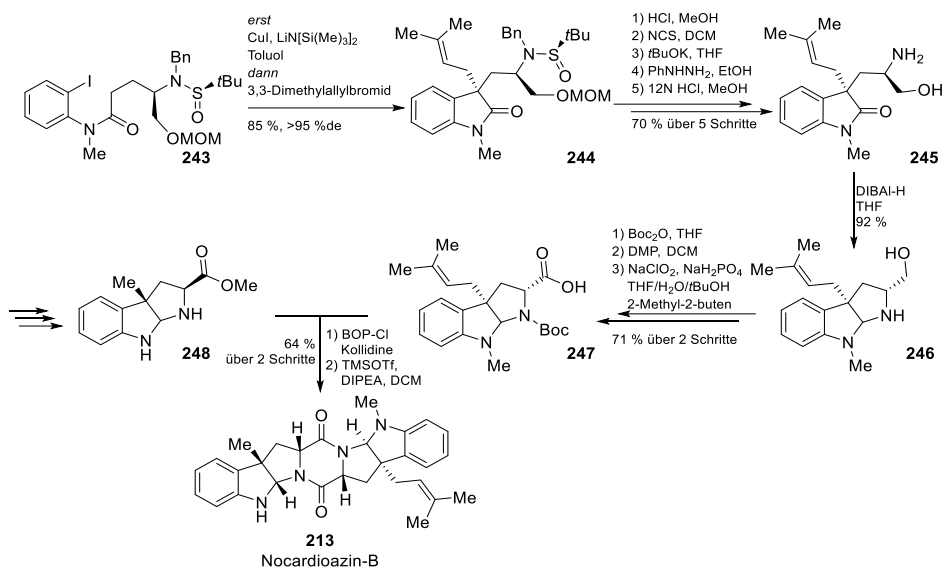
Schema 44: Totalsynthese von Nocardioazin-B ( 213 ) nach Zhang et al. über eine Kupfer-katalysierte sequenzielle Arylierung-Alkylierung ausgehend von \sigma -Haloaniliden. [222]
