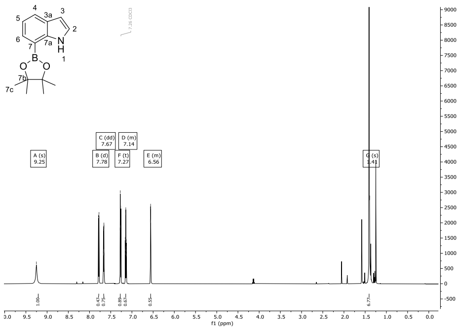
Abbildung 142: 1 H-NMR-Spektrum (600 MHz) von Verbindung 38 in CDCl 3 .
