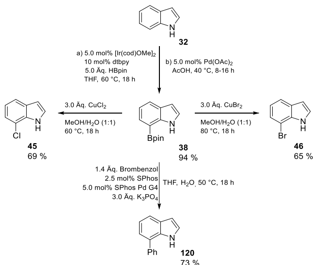
Schema 19: Synthese von 7-Chlor-, 7-Brom- und 7-Phenyl-Indol ( 45 , 46 und 120 ) über die Borylierung nach Movassaghi et al. [84]
