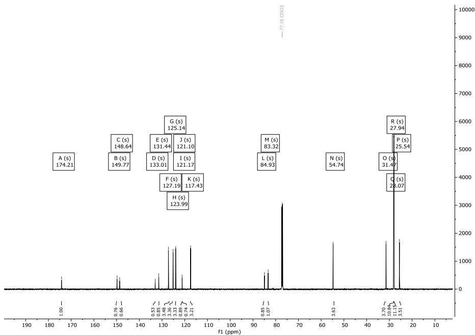
Abbildung 159: ^{13}\text{C} -NMR-Spektrum (151 MHz) von Verbindung 90 in \text{CDCl}_3 .
