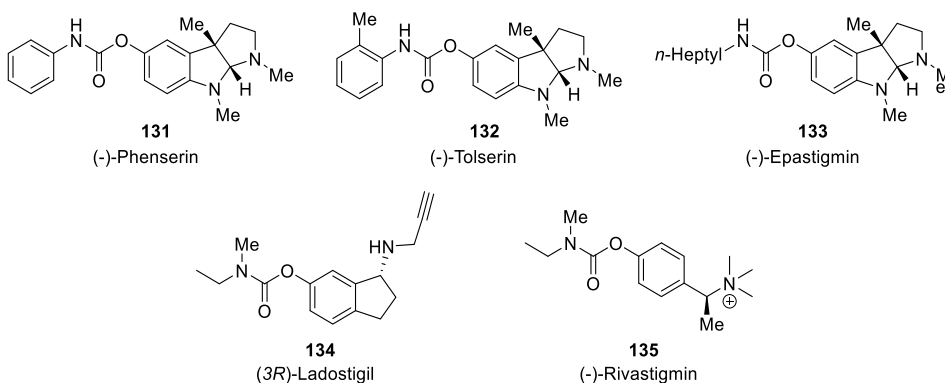
Abbildung 35: Chemische Struktur der synthetischen Physostigmin-Derivate Phenserin, Tolserin und Epastigmin sowie weitere Analoga mit parasympathomimetischer Wirkung.
