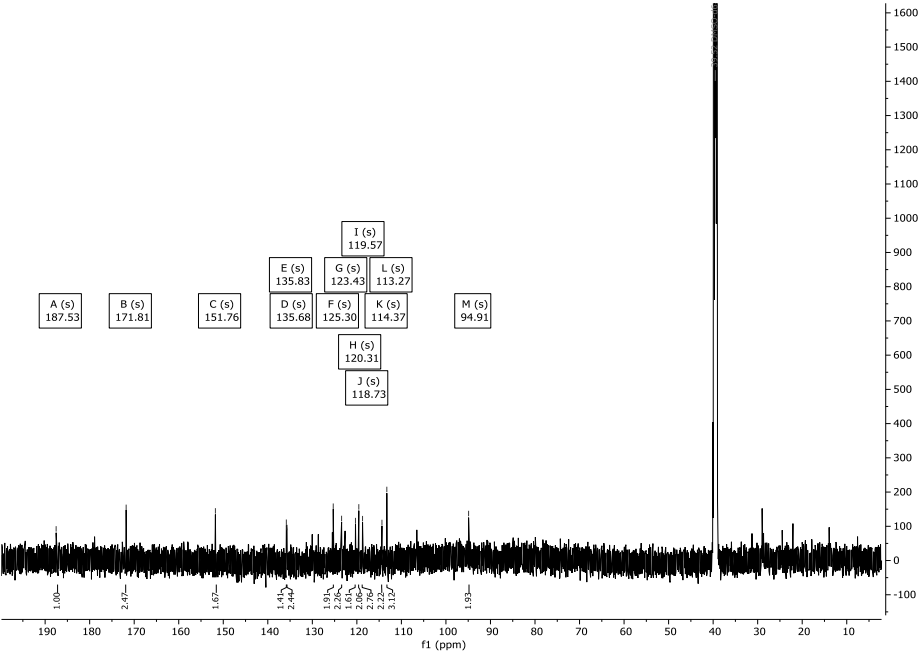
Abbildung 179: 13 C-NMR-Spektrum (151 MHz) der blauen Fraktion von Verbindung 95 in d 6 -DMSO.
