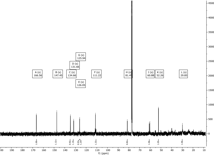
Abbildung 298: ^{13}\text{C} -NMR-Spektrum (76 MHz) von Verbindung 324 in \text{CDCl}_3 .
