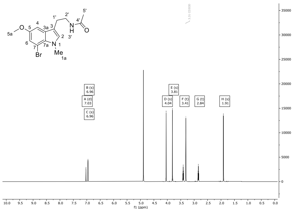
Abbildung 231: ^1\text{H} -NMR-Spektrum (600 MHz) von Verbindung 201 in \text{CD}_3\text{OD} .
