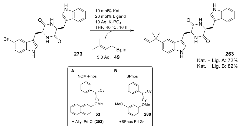
Schema 54: Prenylierung des 5-Brom-DKP 273 zum 5-Prenyl-DKP 263 gemäß der Bedingungen von Reisman et al. [219] und Buchwald et al. [89]
