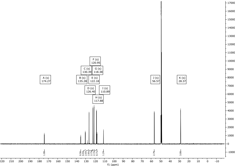
Abbildung 129: ^{13}\text{C} -NMR-Spektrum (151 MHz) von Verbindung 82 in \text{CD}_3\text{OD} .
