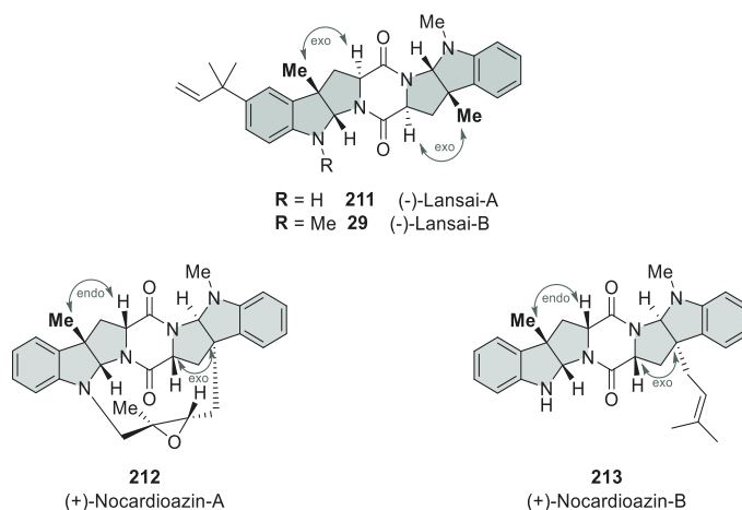
Abbildung 52: Chemische Struktur von (-)-Lansai-A und -B sowie (+)-Nocardioazin-A und -B.
