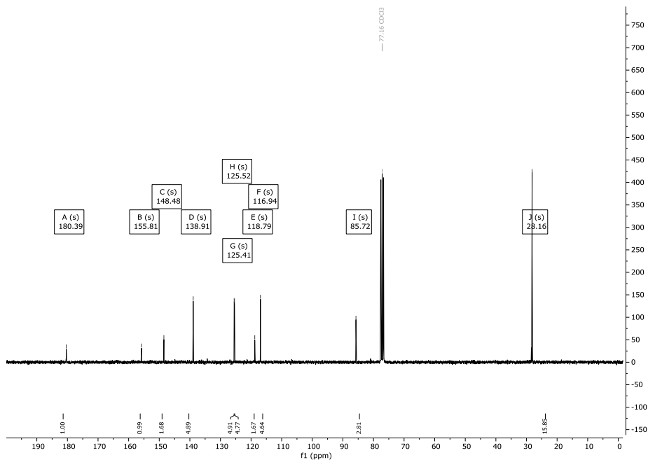
Abbildung 163: ^{13}\text{C} -NMR-Spektrum (151 MHz) von Verbindung 72 in \text{CDCl}_3 .
