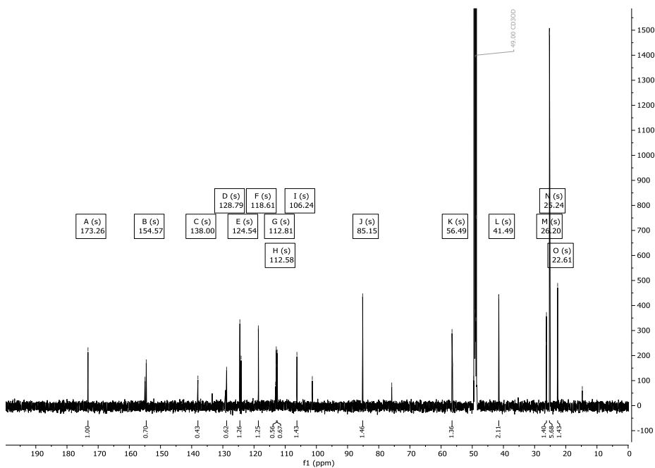
Abbildung 192: ^{13}\text{C} -NMR-Spektrum (151 MHz) von Verbindung 171 in \text{CD}_3\text{OD} .
