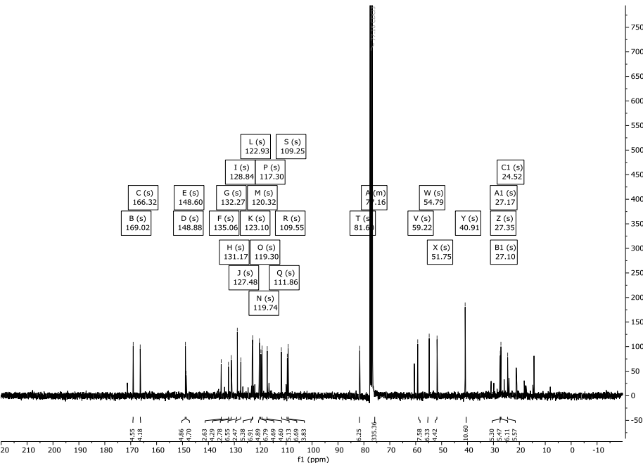
Abbildung 313: ^{13}\text{C} -NMR-Spektrum (76 MHz) von Verbindung 335 in \text{CDCl}_3 .
