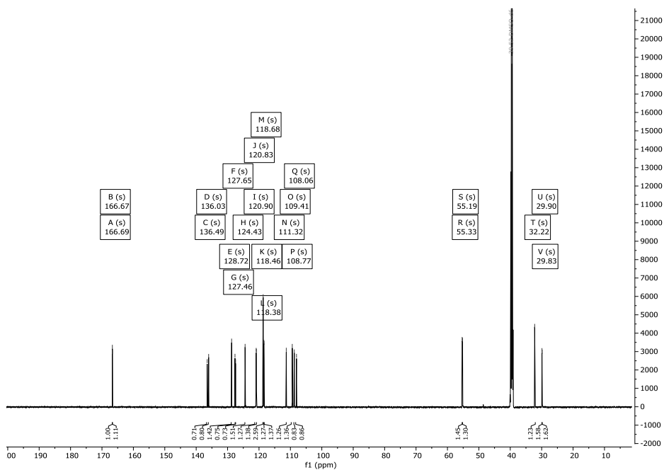
Abbildung 272: ^{13}\text{C} -NMR-Spektrum (151 MHz) von Verbindung 346 in d_6 -DMSO.
