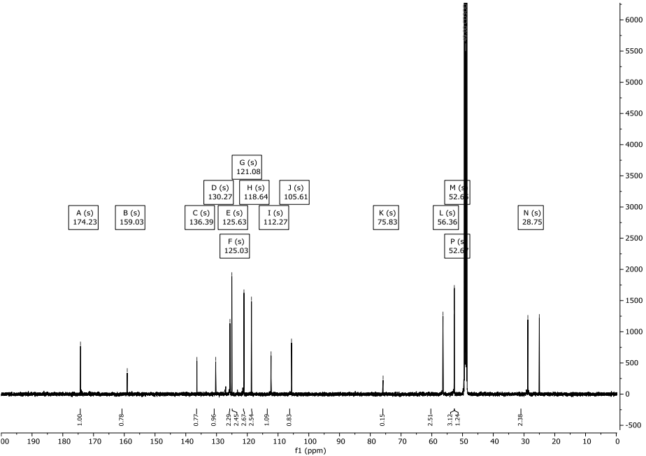
Abbildung 113: 13 C-NMR-Spektrum (151 MHz) von Verbindung 118 in CD 3 OD.
