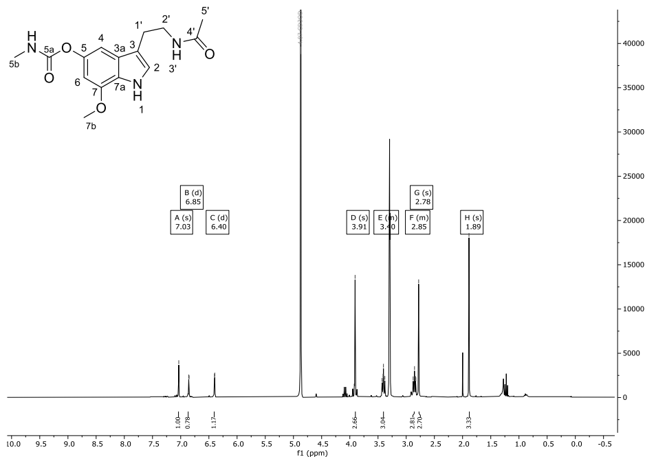
Abbildung 225: ^1\text{H} -NMR-Spektrum (300 MHz) von Verbindung 195 in \text{CD}_3\text{OD} .
