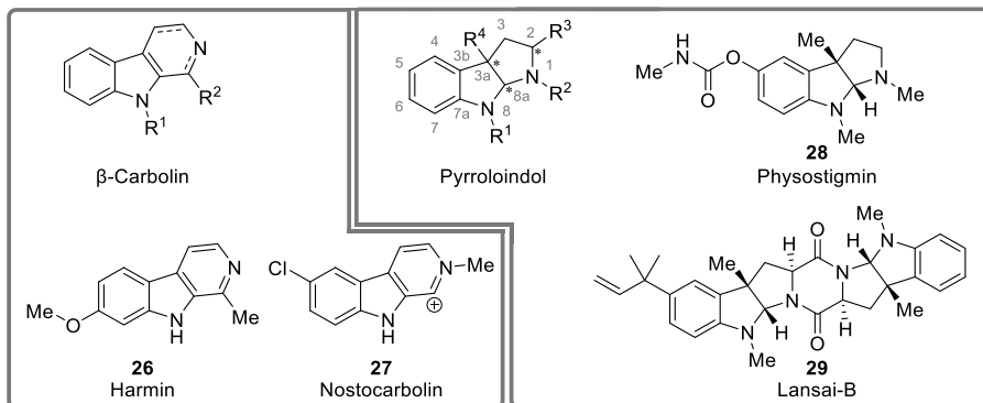
Abbildung 8: Grundstruktur der \beta -Carboline und Pyrroloindole, sowie die chemische Struktur von Harmin ( 26 ), Nostocarbolin ( 27 ), Physostigmin ( 28 ) und Lansai-B ( 29 ).
