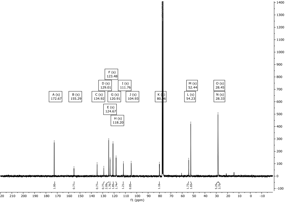
Abbildung 105: ^{13}\text{C} -NMR-Spektrum (76 MHz) von Verbindung 104 in \text{CDCl}_3 .
