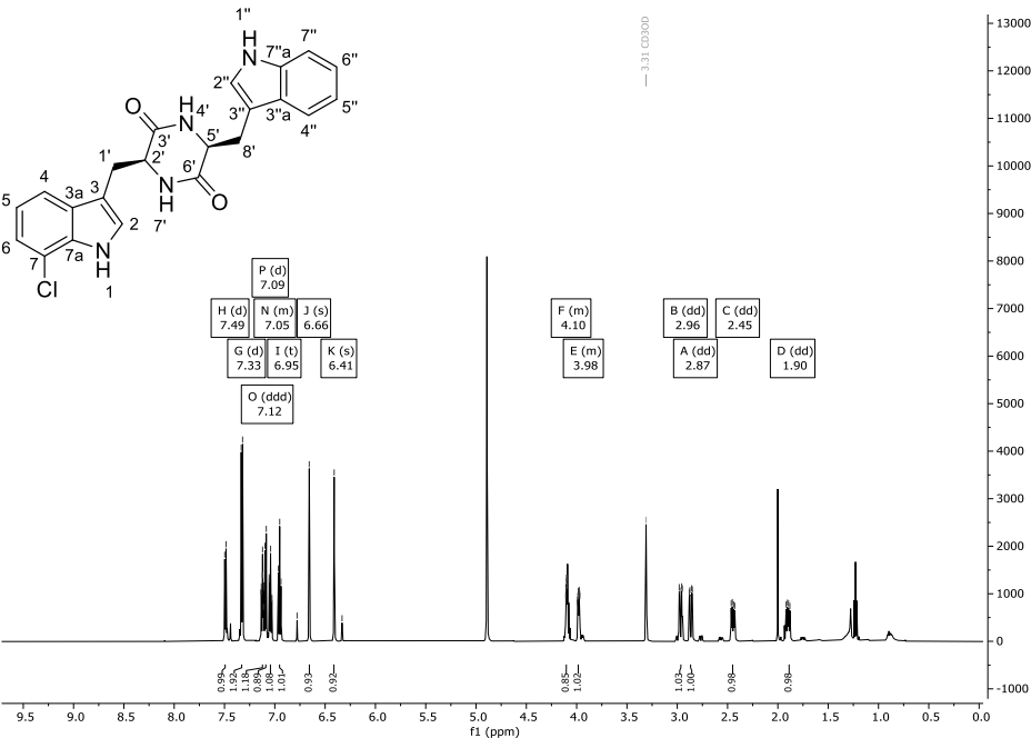
Abbildung 269: 1 H-NMR-Spektrum (600 MHz) von Verbindung 320 in CD 3 OD.
