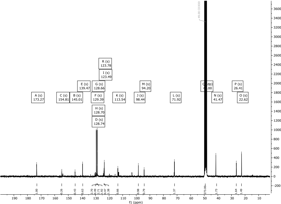
Abbildung 198: 13 C-NMR-Spektrum (151 MHz) von Verbindung 183 in CD 3 OD.
