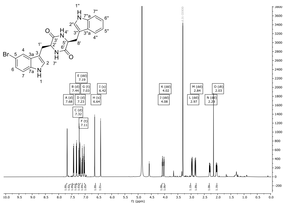
Abbildung 255: ^1\text{H} -NMR-Spektrum (600 MHz) von Verbindung 273 in \text{CD}_3\text{OD} .
