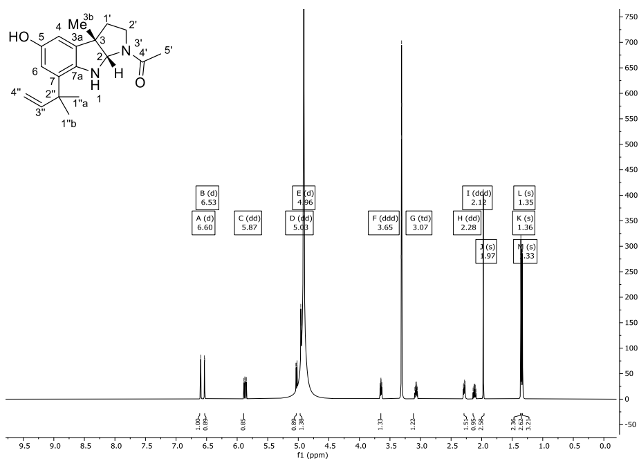
Abbildung 247: Synthetisches ^1\text{H} -NMR-Spektrum (700 MHz) des prädominanten Rotamers von Verbindung 204 in \text{CD}_3\text{OD} .
