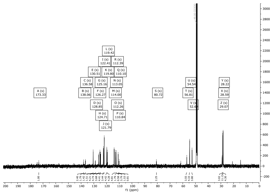
Abbildung 252: ^{13}\text{C} -NMR-Spektrum (151 MHz) von Verbindung 286 in \text{CD}_3\text{OD} .
