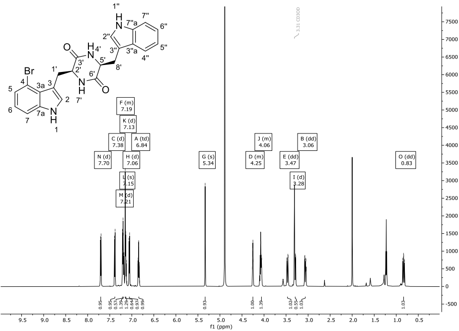
Abbildung 257: 1 H-NMR-Spektrum (600 MHz) von Verbindung 313 in CD 3 OD.
