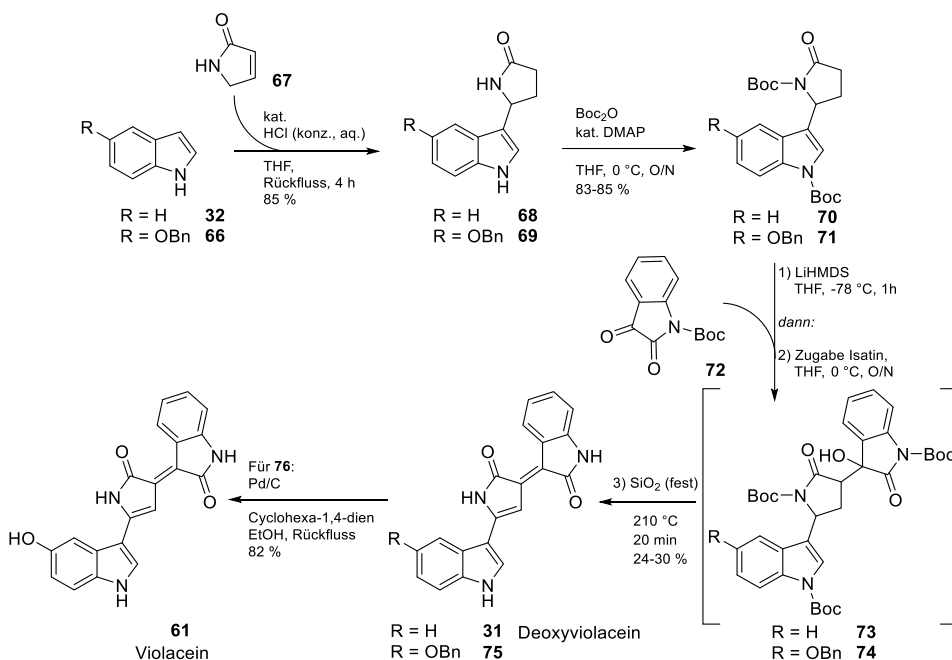
Schema 9: Totalsynthese von Violacein ( 61 ) und Deoxyviolacein ( 31 ) nach Wille und Steglich über eine Aldol-Kondensation ausgehend von Indol ( 32 ). [104]
