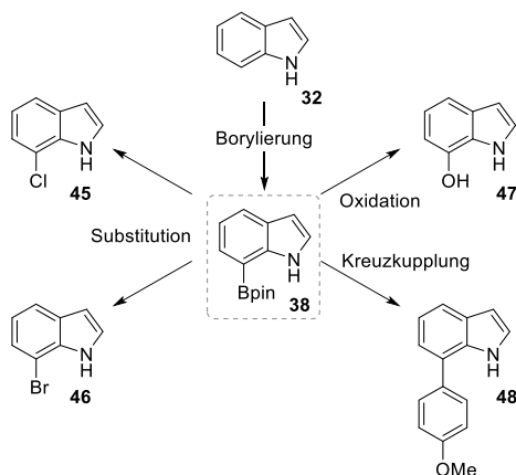
Schema 3: Schematische Darstellung der Möglichkeiten zur Derivatisierung von Indol ( 32 ) durch Borylierung. [84]
