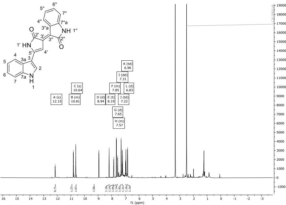
Abbildung 168: 1 H-NMR-Spektrum (600 MHz) der violetten Fraktion von Verbindung 31 in d 6 -DMSO.
