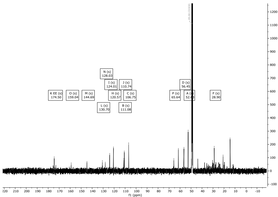
Abbildung 115: ^{13}\text{C} -NMR-Spektrum (151 MHz) von Verbindung 117 in \text{CD}_3\text{OD} .
