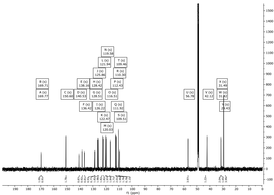
Abbildung 307: ^{13}\text{C} -NMR-Spektrum (151 MHz) von Verbindung 263 in \text{CD}_3\text{OD} .
