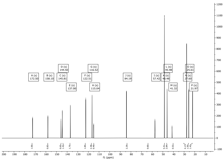
Abbildung 236: Synthetisches ^{13}\text{C} -NMR-Spektrum (151 MHz) des geringer-vorliegendes Rotamers von Verbindung 196 in \text{CD}_3\text{OD} .
