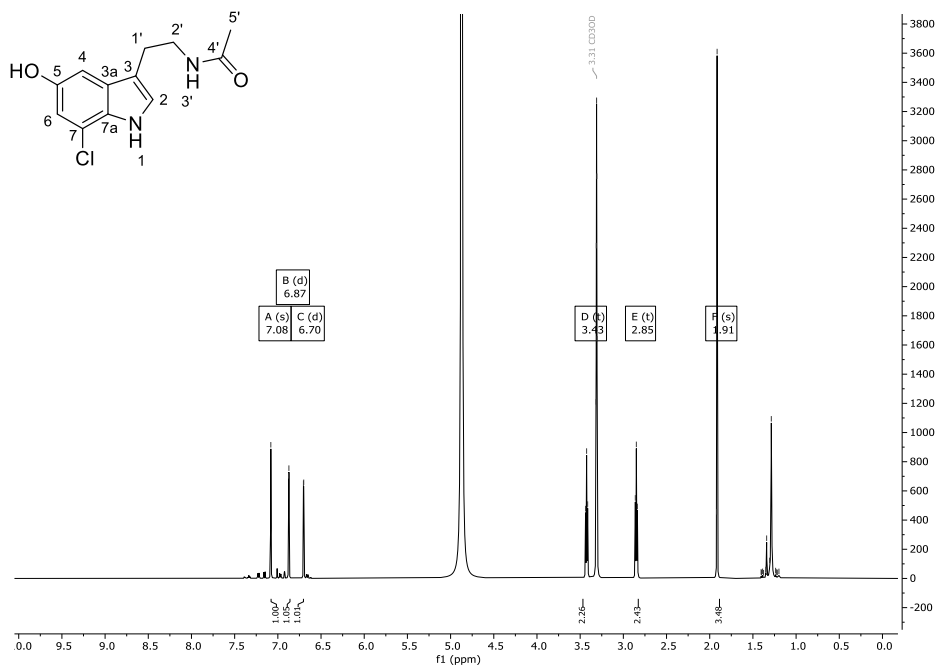
Abbildung 213: ^1\text{H} -NMR-Spektrum (600 MHz) von Verbindung 176 in \text{CDCl}_3 .
