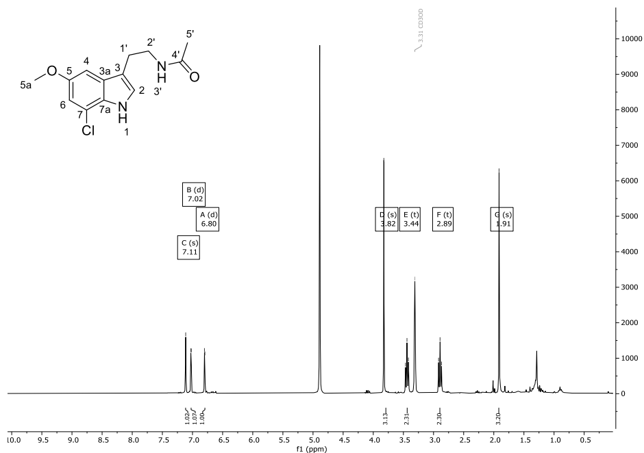
Abbildung 203: 1 H-NMR-Spektrum (600 MHz) von Verbindung 173 in CD 3 OD.
