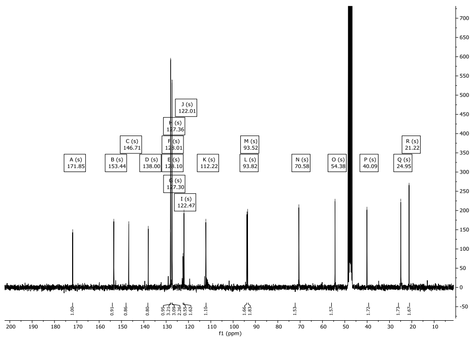
Abbildung 200: ^{13}\text{C} -NMR-Spektrum (151 MHz) von Verbindung 193 in \text{CD}_3\text{OD} .
