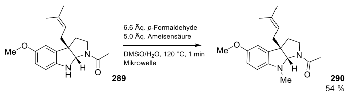
Schema 56: N-Methylierung des Modells substrats 289 unter Eschweiler-Clarke Bedingungen in einer reduktiven Aminierung. [236]
