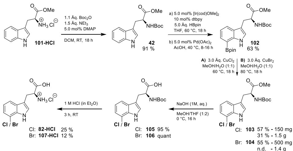
Schema 13: Synthese von 7-Chlor und 7-Bromtryptophan 82 und 107 über die Borylierungs/Protodeborylierungs-Sequenz nach Movassaghi et al. mit anschließender Chlorierung bzw. Bromierung und Entfernung der PGs.
