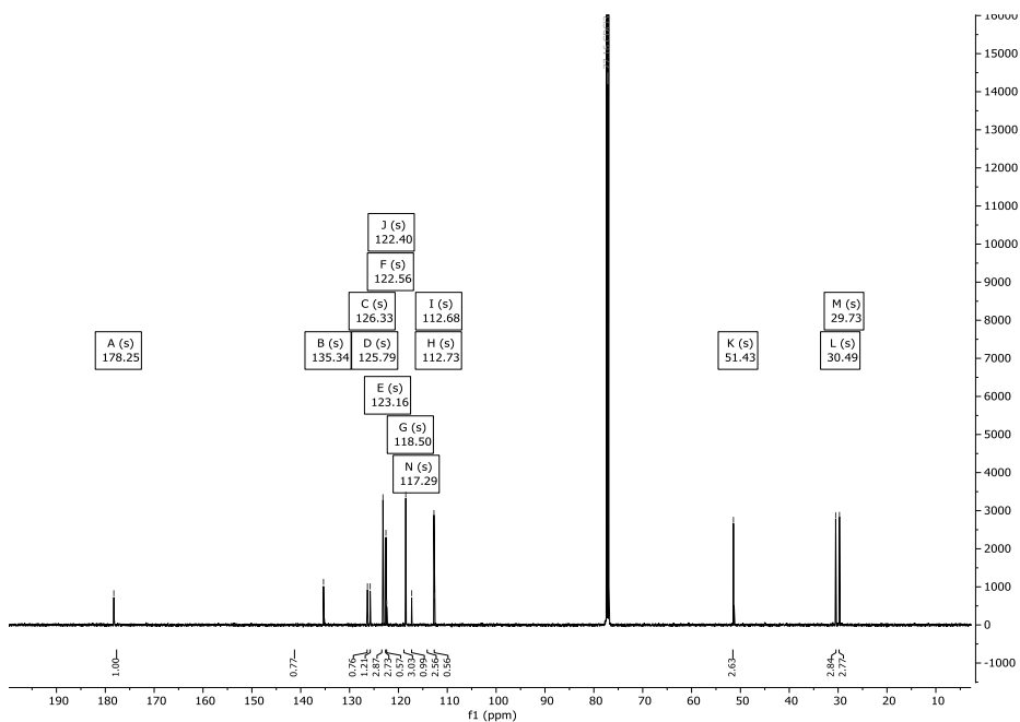
Abbildung 155: ^{13}\text{C} -NMR-Spektrum (151 MHz) von Verbindung 87 in \text{CDCl}_3 .
