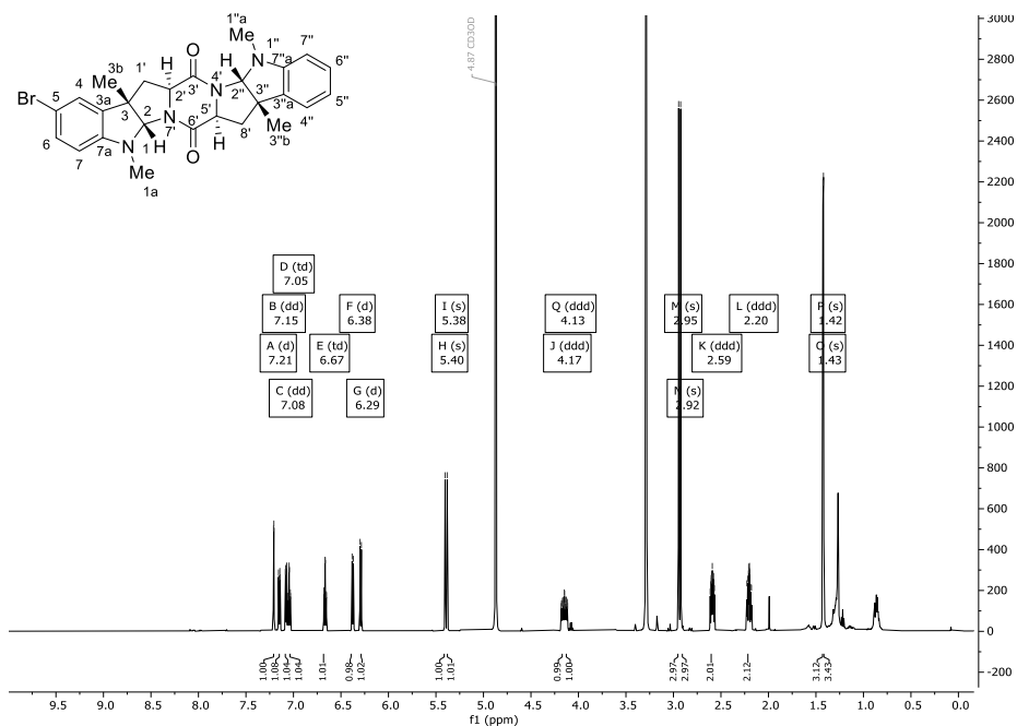
Abbildung 318: ^1\text{H} -NMR-Spektrum (600 MHz) von Verbindung 293 in \text{CD}_3\text{OD} .
