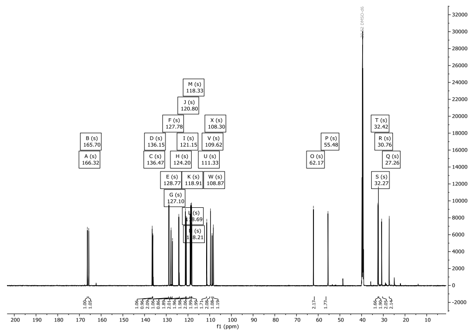
Abbildung 274: 13 C-NMR-Spektrum (151 MHz) von Verbindung 347 in d 6 -DMSO.
