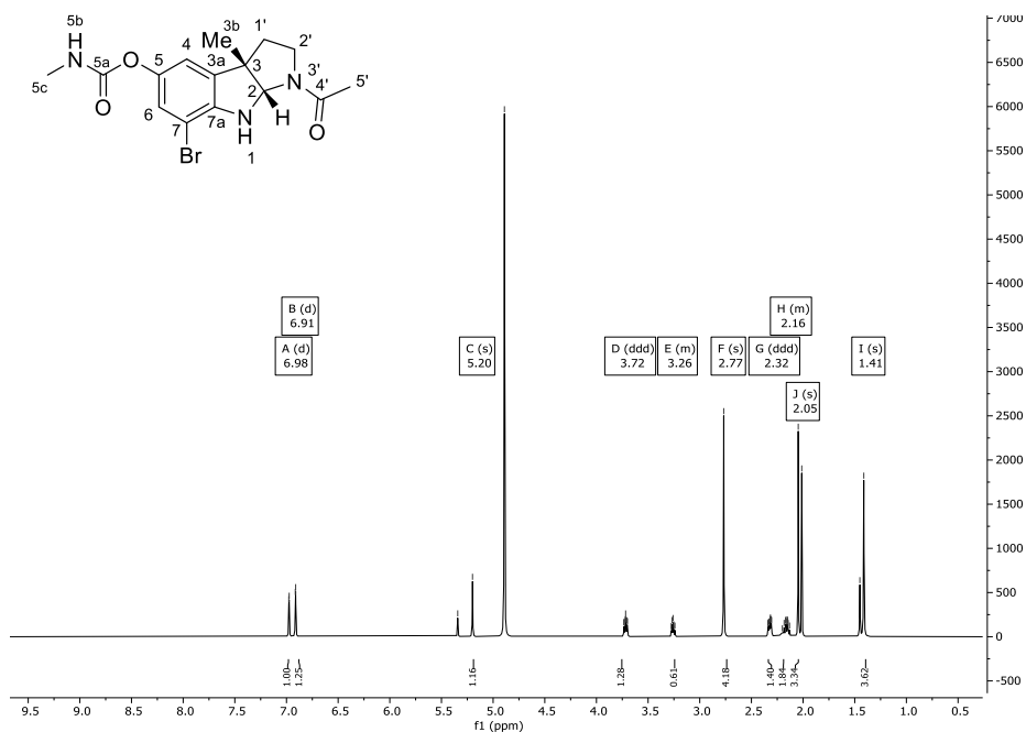
Abbildung 239: Synthetisches ^1\text{H} -NMR-Spektrum (600MHz) des prädominanten Rotamers von Verbindung 197 in \text{CD}_3\text{OD} .
