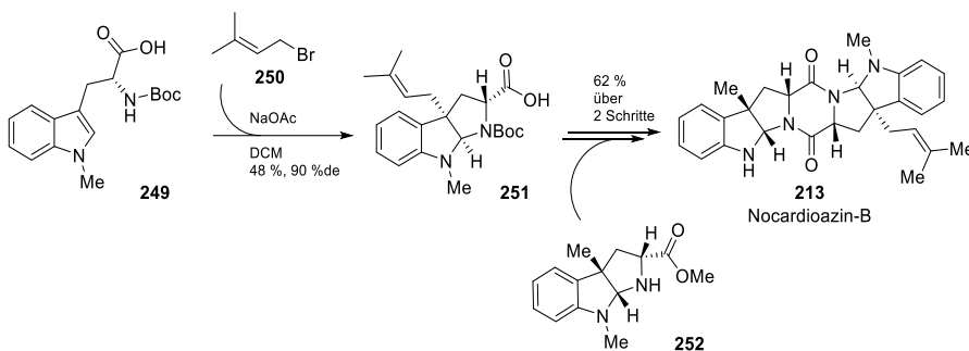
Schema 45: Biomimetische Totalsynthese von Nocardioazin-B nach Viswanathan et al. mit der C3 -Prenylierung als Schlüsselschritt. [223]
