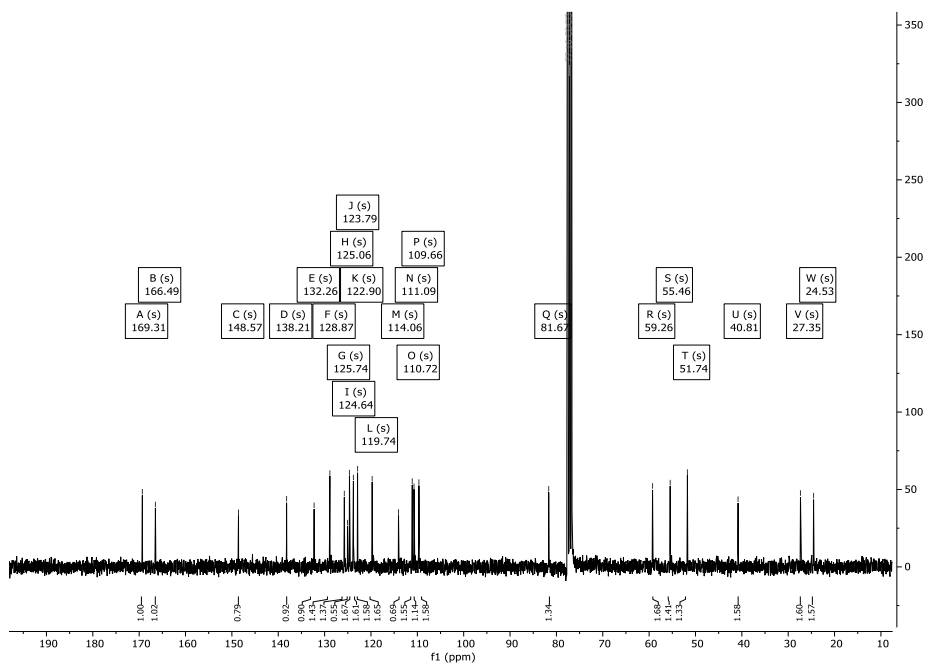
Abbildung 288: ^{13}\text{C} -NMR-Spektrum (76 MHz) von Verbindung 331 in \text{CDCl}_3 .
