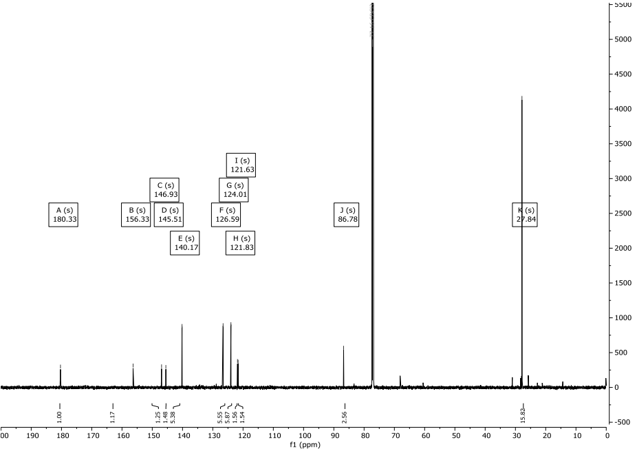
Abbildung 165: ^{13}\text{C} -NMR-Spektrum (151 MHz) von Verbindung 94 in \text{CDCl}_3 .
