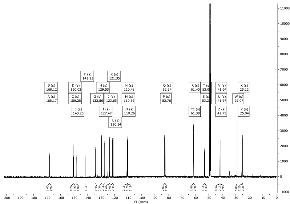
Abbildung 309: ^{13}\text{C} -NMR-Spektrum (151 MHz) von Verbindung 281 in \text{CD}_3\text{OD} .
