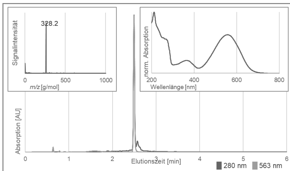
Abbildung 31: Chromatogramm des synthetisierten dVio ( 31 ) in der hier verwendeten LC-MS-Methode (Atlantis T3 mit Wasser/Acetonitril (5 % – 80 %) + Ameisensäure (0.1 %)). Aufgetragen ist die Absorption bei 280 nm (blau) und 563 nm (orange) gegen die Elutionszeit. Für den Peak bei ca. 2.5 min ist zusätzlich das Massenspektrum (Signalintensität gegen Molekülmasse, oben-links) sowie das Absorptionsspektrum (Absorption gegen die Wellenlänge, oben-rechts) dargestellt.
