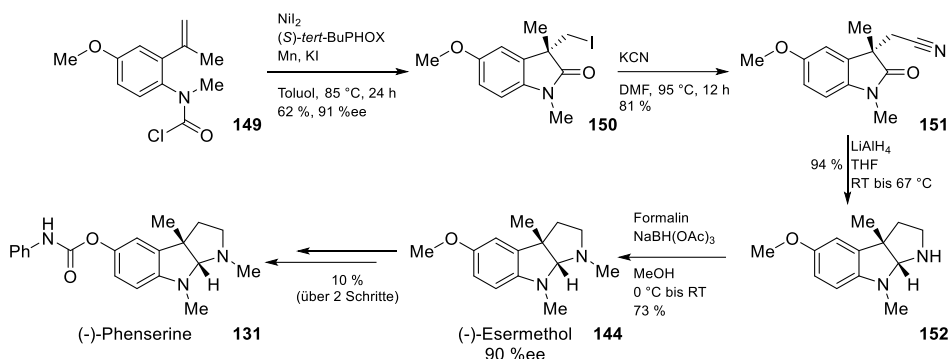
Schema 25: Nickelkatalysierte Synthese von Esermethol ( 144 ) und Phenserine ( 131 ) mittels enantioselektiver Carbamoyl-Iodierung nach Lautens et al. [183]
