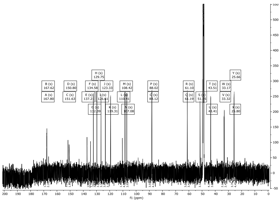
Abbildung 319: ^{13}\text{C} -NMR-Spektrum (151 MHz) von Verbindung 293 in \text{CD}_3\text{OD} .
