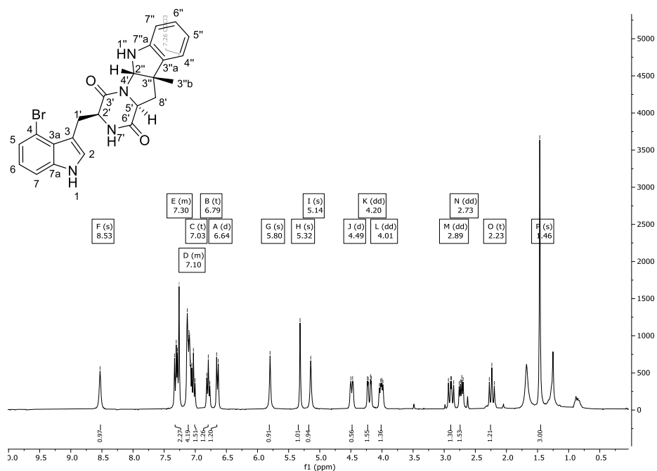
Abbildung 287: ^1\text{H} -NMR-Spektrum (300 MHz) von Verbindung 331 in \text{CDCl}_3 .
