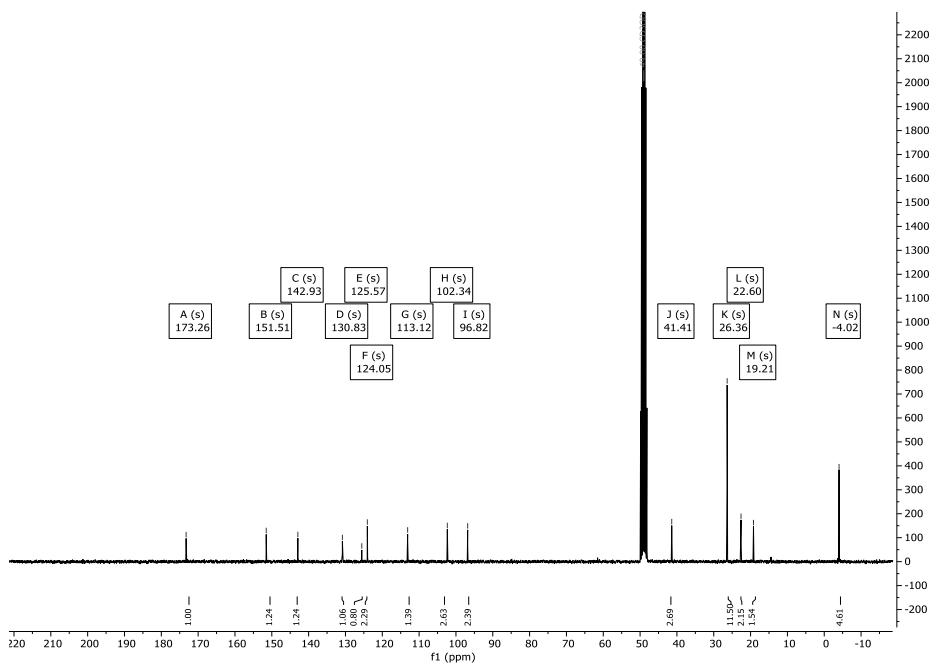
Abbildung 220: ^{13}\text{C} -NMR-Spektrum (151 MHz) von Verbindung 186 in \text{CD}_3\text{OD} .
