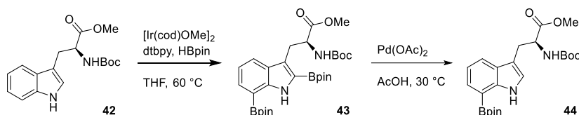
Schema 2: Selektive Borylierung in 7-Position des Indols durch sequenzielle 2,7-Diborylierung mit anschließender Protodeborylierung in 2-Position nach Movassaghi et al. [84]
