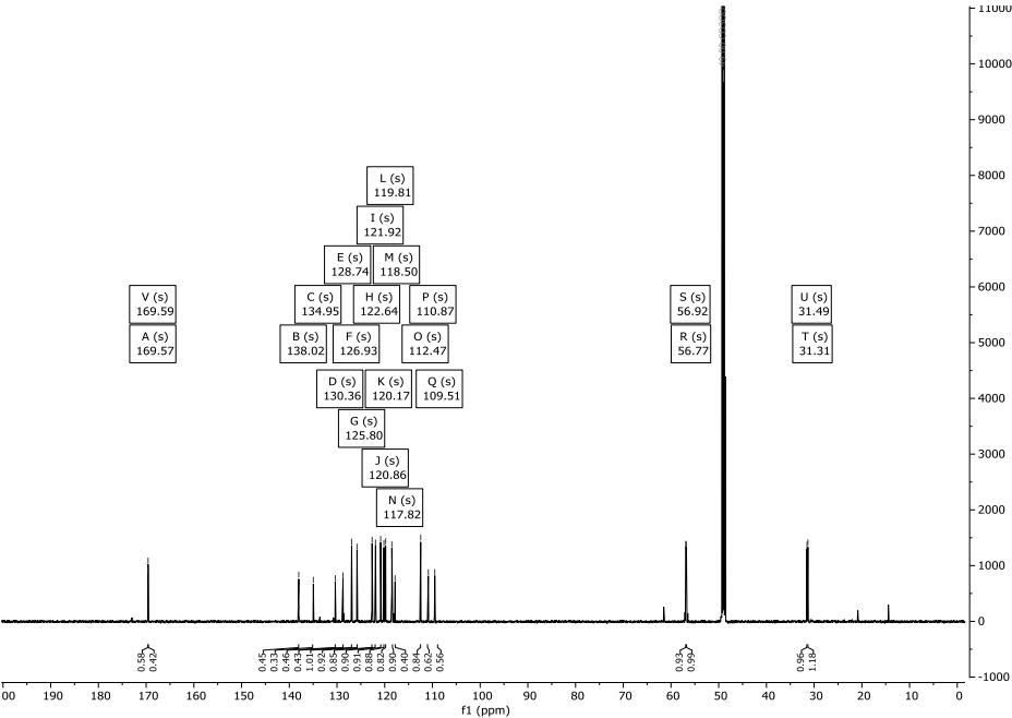
Abbildung 270: 13 C-NMR-Spektrum (151 MHz) von Verbindung 320 in CD 3 OD.
