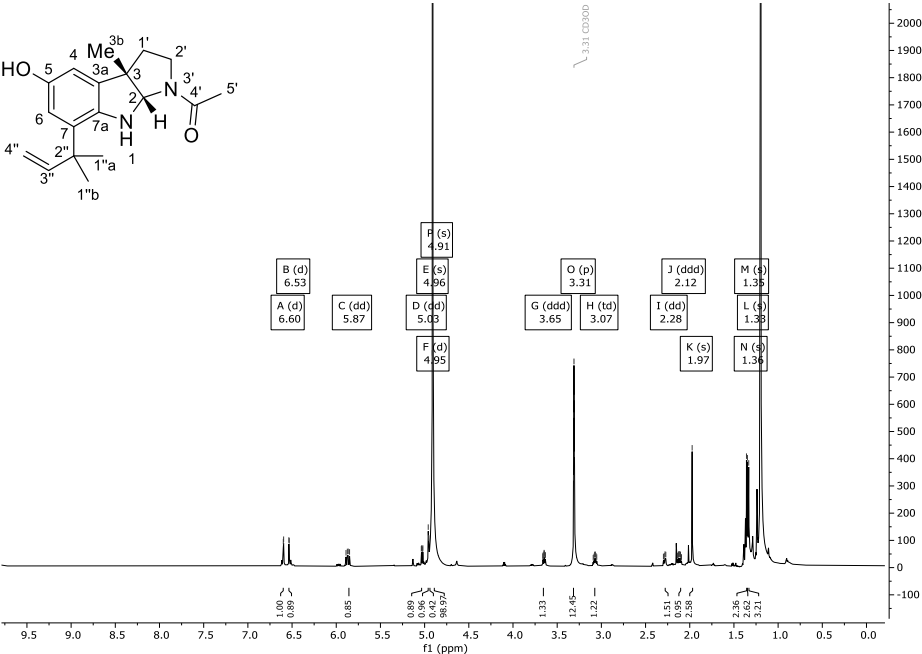
Abbildung 245: ^1\text{H} -NMR-Spektrum (700 MHz) von Verbindung 204 in \text{CD}_3\text{OD} .
