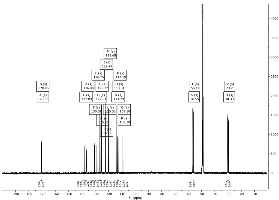
Abbildung 260: 13 C-NMR-Spektrum (151 MHz) von Verbindung 274 in CD 3 OD.
