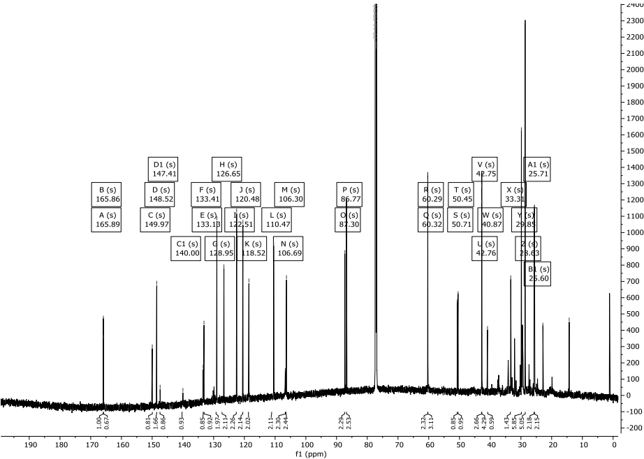
Abbildung 325: 13 C-NMR-Spektrum (176 MHz) von Verbindung 29 in CD 3 OD.
