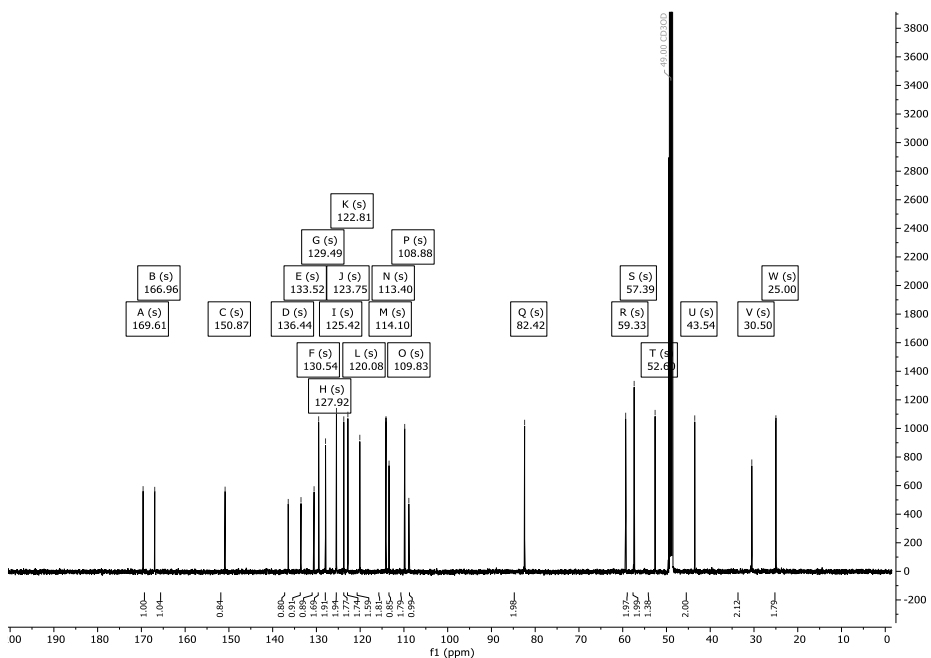
Abbildung 292: ^{13}\text{C} -NMR-Spektrum (151 MHz) von Verbindung 288 in \text{CD}_3\text{OD} .
