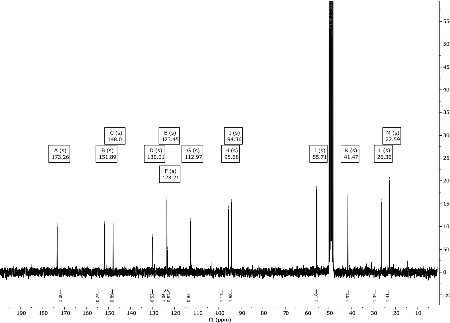
Abbildung 218: ^{13}\text{C} -NMR-Spektrum (151 MHz) von Verbindung 194 in \text{CD}_3\text{OD} .
