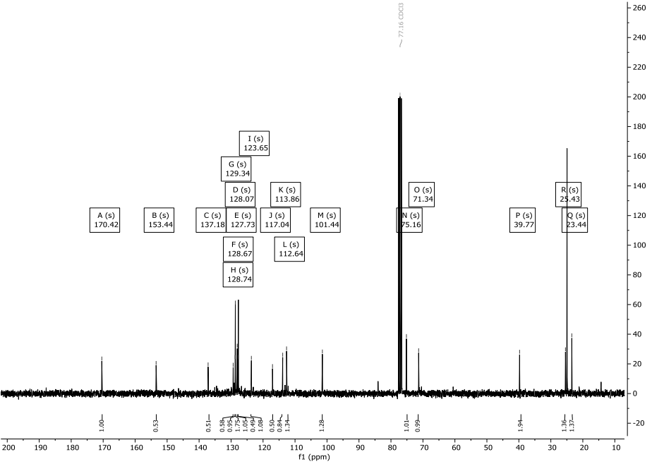
Abbildung 194: 13 C-NMR-Spektrum (151 MHz) von Verbindung 172 in CDCl 3 .
