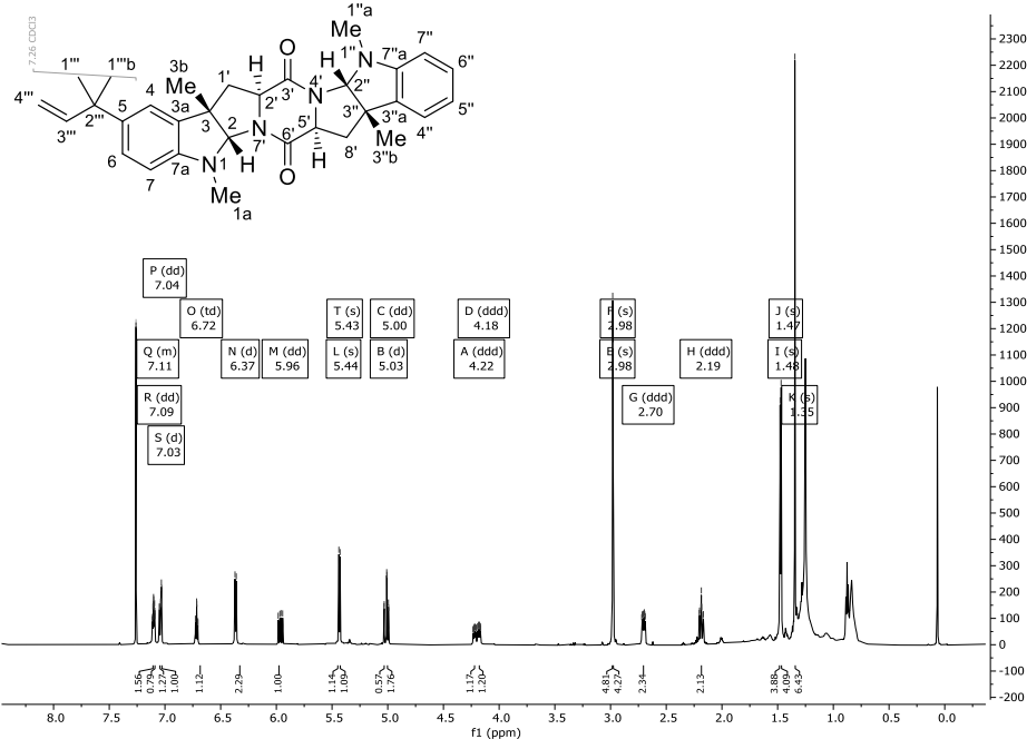
Abbildung 324: 1 H-NMR-Spektrum (700 MHz) von Verbindung 29 in CDCl 3 .
