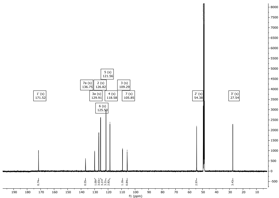
Abbildung 123: 13 C-NMR-Spektrum (151 MHz) von Verbindung 107-HCl in CD 3 OD.
