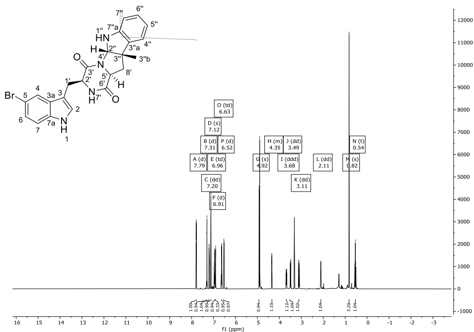
Abbildung 291: ^1\text{H} -NMR-Spektrum (600 MHz) von Verbindung 288 in \text{CD}_3\text{OD} .
