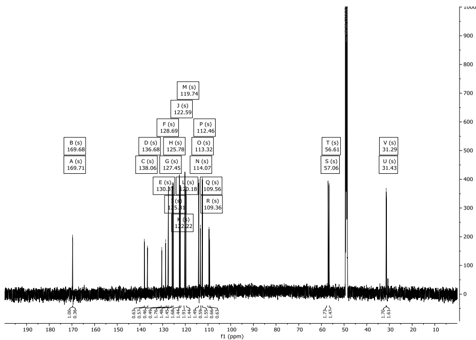
Abbildung 256: ^{13}\text{C} -NMR-Spektrum (151 MHz) von Verbindung 273 in \text{CD}_3\text{OD} .
