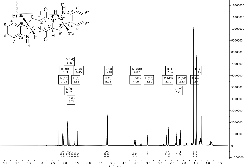
Abbildung 289: ^1\text{H} -NMR-Spektrum (900 MHz) von Verbindung 322 in \text{CDCl}_3 .
