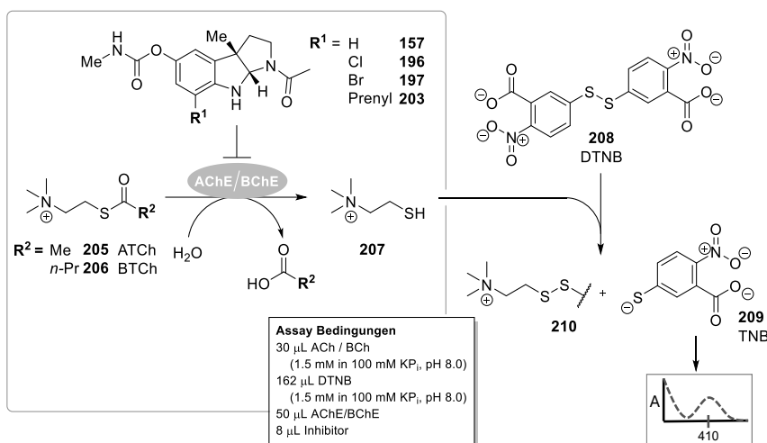
Abbildung 44: Schematische Darstellung des Ellmans-Assays, bei dem die Inhibition der AChE/BChE durch die HHP-Verbindungen 157 , 196 , 197 und 203 untersucht wird. Die Enzyme katalysieren die Hydrolyse von Acetyl- und Butyrylthiocholin ( 205/206 ) zu Thiocholin ( 207 ), welches die Disulfidbrücke des DTNB ( 208 ) spaltet. Die resultierende Freisetzung von TNB ( 209 ) kann anhand der Absorption bei 412 nm quantitativ gemessen werden. [206]
