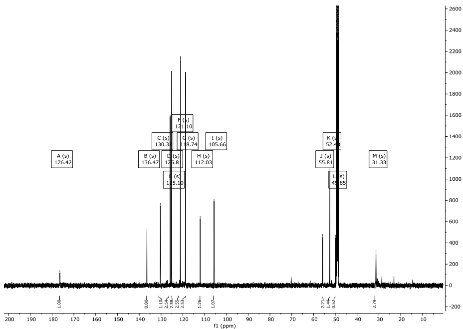
Abbildung 131: 13 C-NMR-Spektrum (151 MHz) von Verbindung 294 in CD 3 OD.
