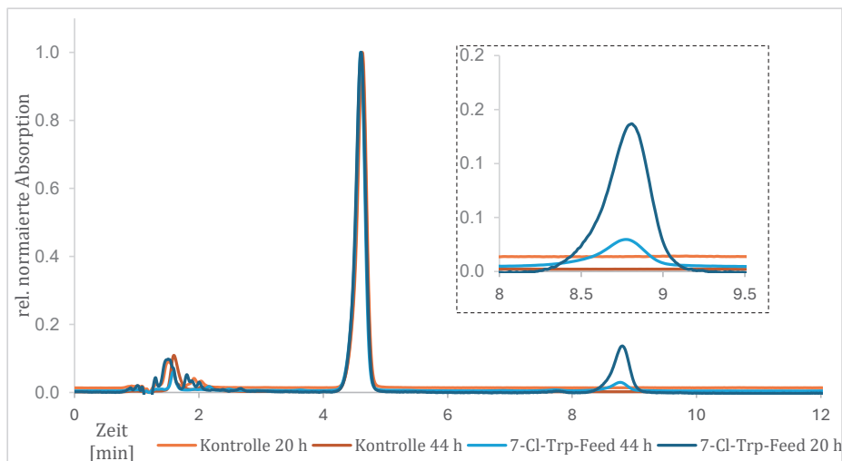
Abbildung 27: Überlagertes Chromatogramm der Mutasynthese-Ansätze in LB-Medium nach 19 h oder 44 h bei der etablierten HPLC-Methode (Isaspher C18-Säule mit Wasser/Acetonitril: 55/45). Aufgetragen ist die Absorption (normiert auf den höchsten Absorptionswert) bei der maximalen Absorptionswellenlänge gegen die Elutionszeit. In hell-/dunkelblau sind die Ansätze mit zugefüttertem 7-Chlor-Tryptophan ( 82 – 1 mM) dargestellt, in orange/rot die Kontrollgruppen ohne Trp-Zusatz. Der Bereich von 8 – 9.5 min ist noch einmal vergrößert abgebildet.
