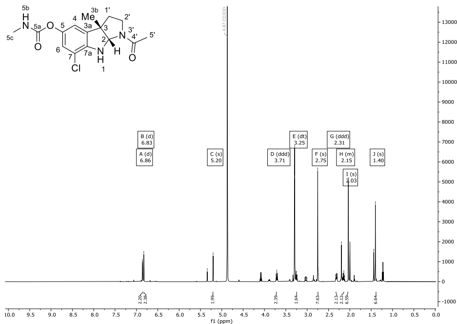
Abbildung 233: ^1\text{H} -NMR-Spektrum (600 MHz) von Verbindung 196 in \text{CD}_3\text{OD} .
