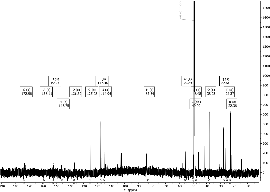
Abbildung 238: ^{13}\text{C} -NMR-Spektrum (151 MHz) von Verbindung 197 in \text{CD}_3\text{OD} .
