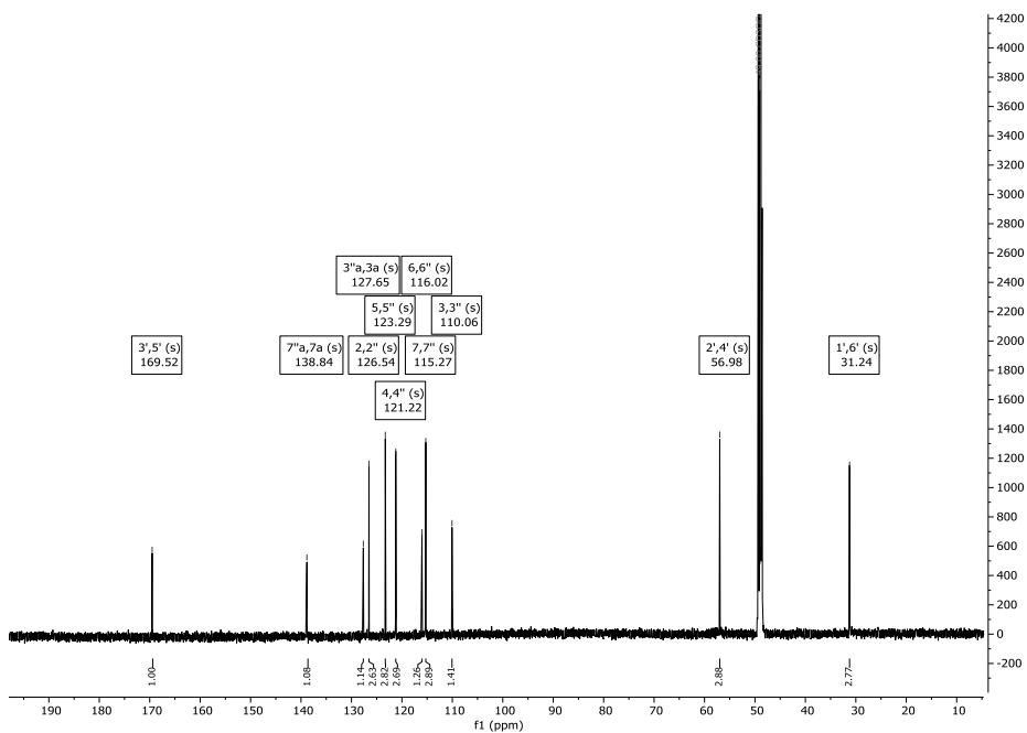
Abbildung 280: ^{13}\text{C} -NMR-Spektrum (151 MHz) von Verbindung 317 in \text{CD}_3\text{OD} .
