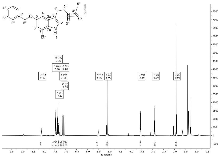
Abbildung 195: ^1\text{H} -NMR-Spektrum (600 MHz) von Verbindung 174 in \text{CDCl}_3 .
