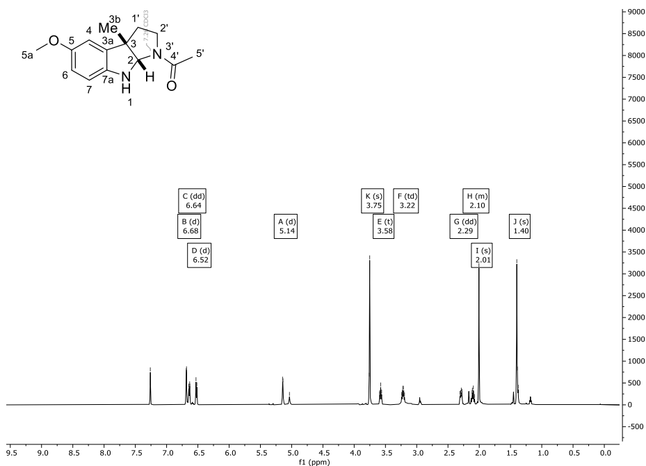
Abbildung 227: ^1\text{H} -NMR-Spektrum (600 MHz) von Verbindung rac -200 in \text{CDCl}_3 .
