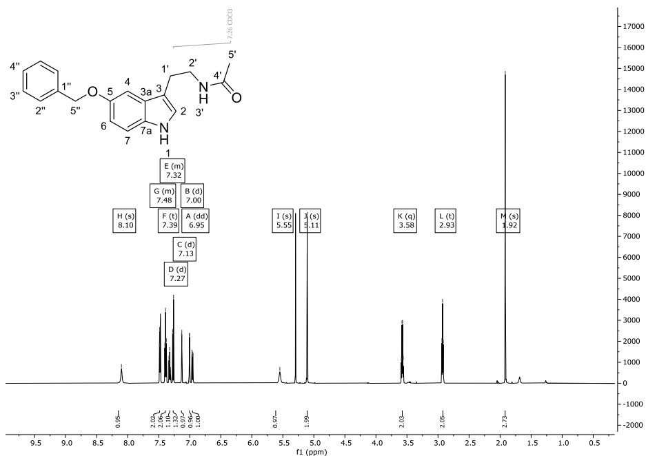
Abbildung 187: ^{13}\text{C} -NMR-Spektrum (151 MHz) von Verbindung 161 in \text{CDCl}_3 .
