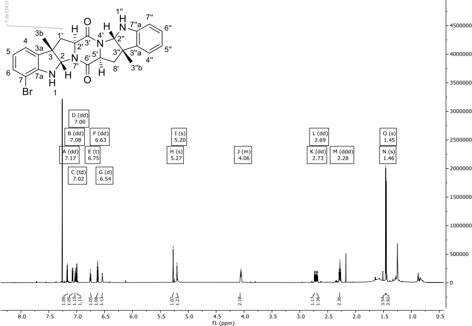
Abbildung 301: ^1\text{H} -NMR-Spektrum (900 MHz) von Verbindung 327 in \text{CDCl}_3 .
