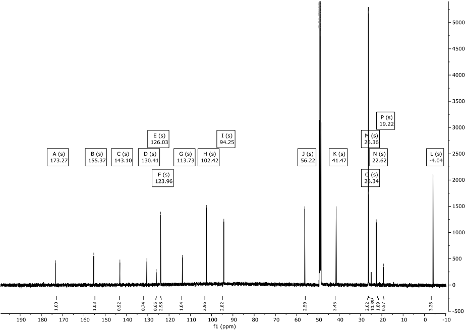
Abbildung 210: 13 C-NMR-Spektrum (151 MHz) von Verbindung 184 in CD 3 OD.
