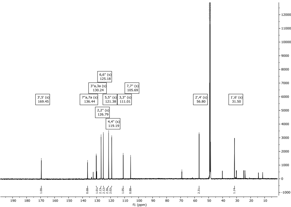
Abbildung 282: ^{13}\text{C} -NMR-Spektrum (151 MHz) von Verbindung 319 in \text{CD}_3\text{OD} .
