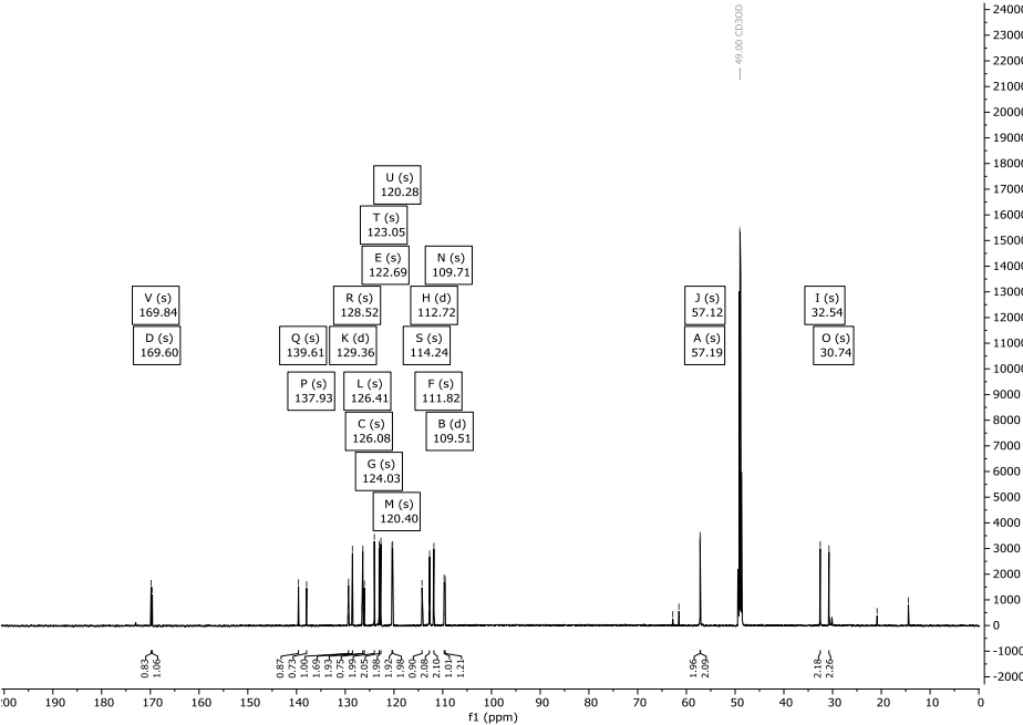
Abbildung 258: 13 C-NMR-Spektrum (151 MHz) von Verbindung 313 in CD 3 OD.
