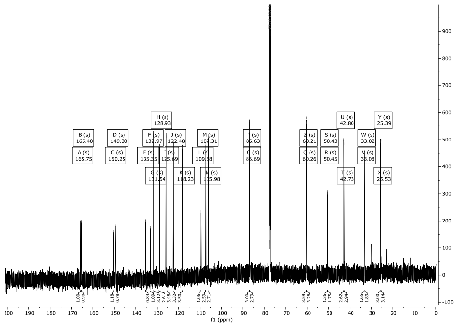
Abbildung 321: ^{13}\text{C} -NMR-Spektrum (151 MHz) von Verbindung 293 in \text{CDCl}_3 .
