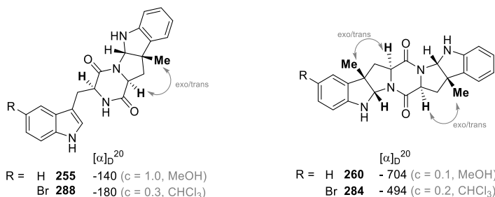
Abbildung 58: Gemessene Drehwerte der bromierten Verbindungen 284 und 288 im Vergleich zu den unsubstituierten Verbindungen 255 und 260 , welche von M. Haase beschrieben wurden. [230]
