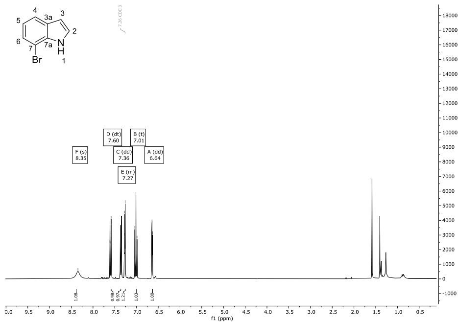
Abbildung 146: ^1\text{H} -NMR-Spektrum (300 MHz) von Verbindung 46 in \text{CDCl}_3 .
