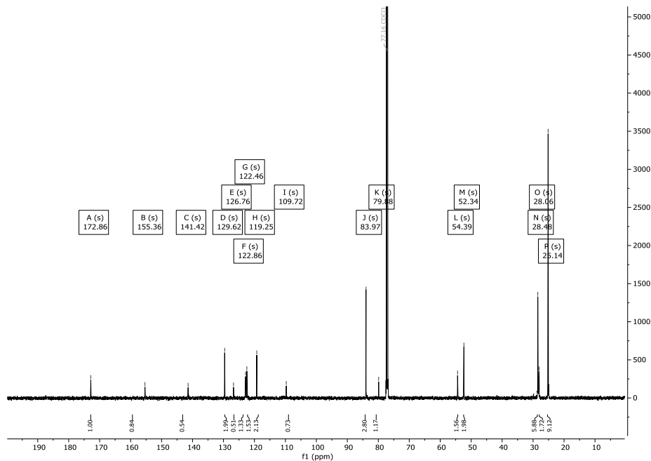
Abbildung 97: ^{13}\text{C} -NMR-Spektrum (151 MHz) von Verbindung 102 in \text{CDCl}_3 .
