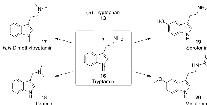
Abbildung 6: Chemische Struktur Tryptamin-artiger Alkaloide wie N,N -Dimethyltryptamin ( 17 ), Gramin ( 18 ), Serotonin ( 19 ) und Melatonin ( 20 ).
